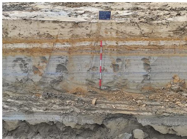
Trincea di scavo - parete W. Colonna stratigrafica 23 (presa da E)
