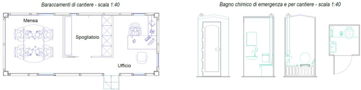
Figura 21: pianta locale baraccamenti e bagni
