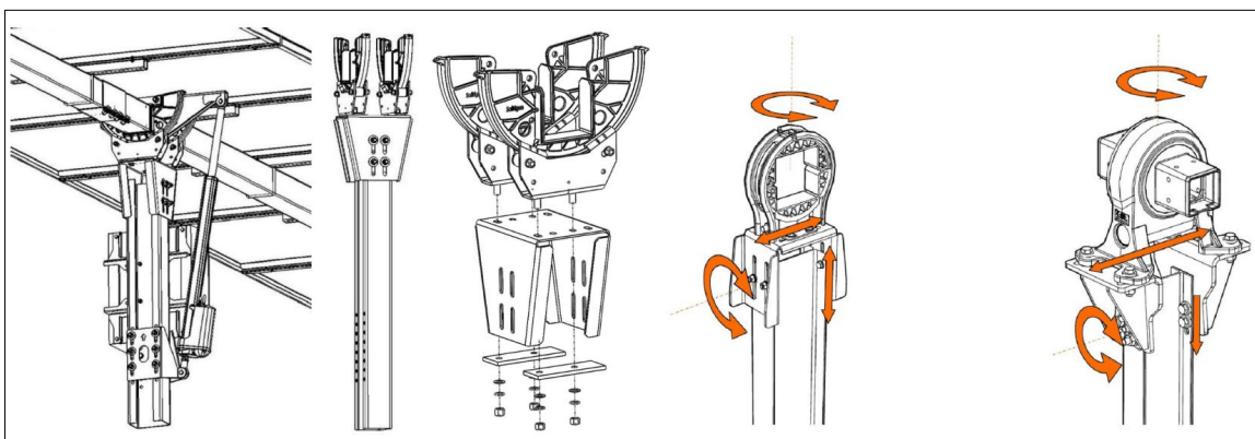
Figura 23: Dettaglio di costruzione delle strutture
