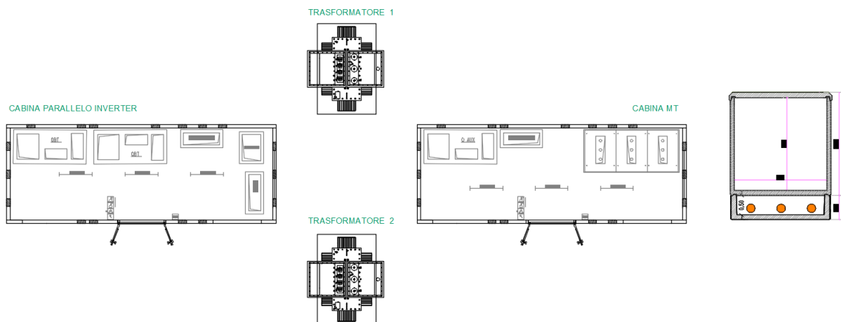
Figura 12: power station a 2 trasformatori
