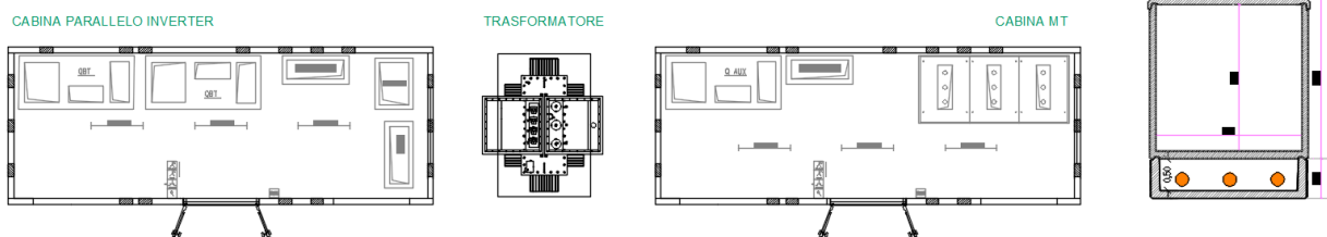
Figura 11: power station ad 1 trasformatore
