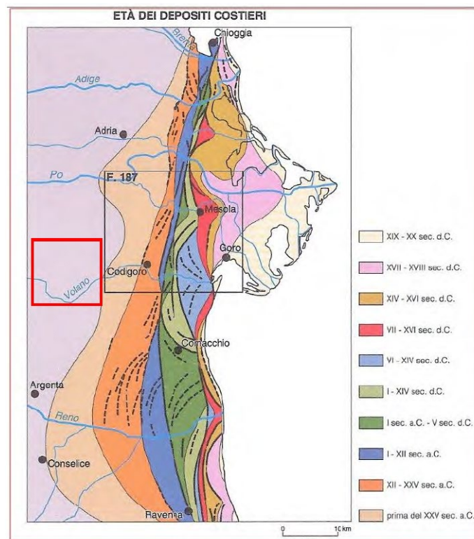
Figura 18: Età dei depositi dell'attuale sistema costiero.
