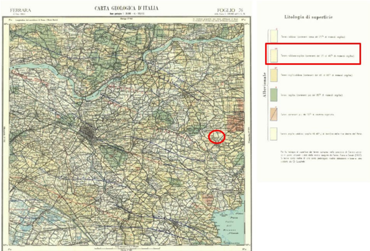
Figura 17 Inquadramento dell'area di intervento sulla Carta Geologica d'Italia in scala a 1:100000.
