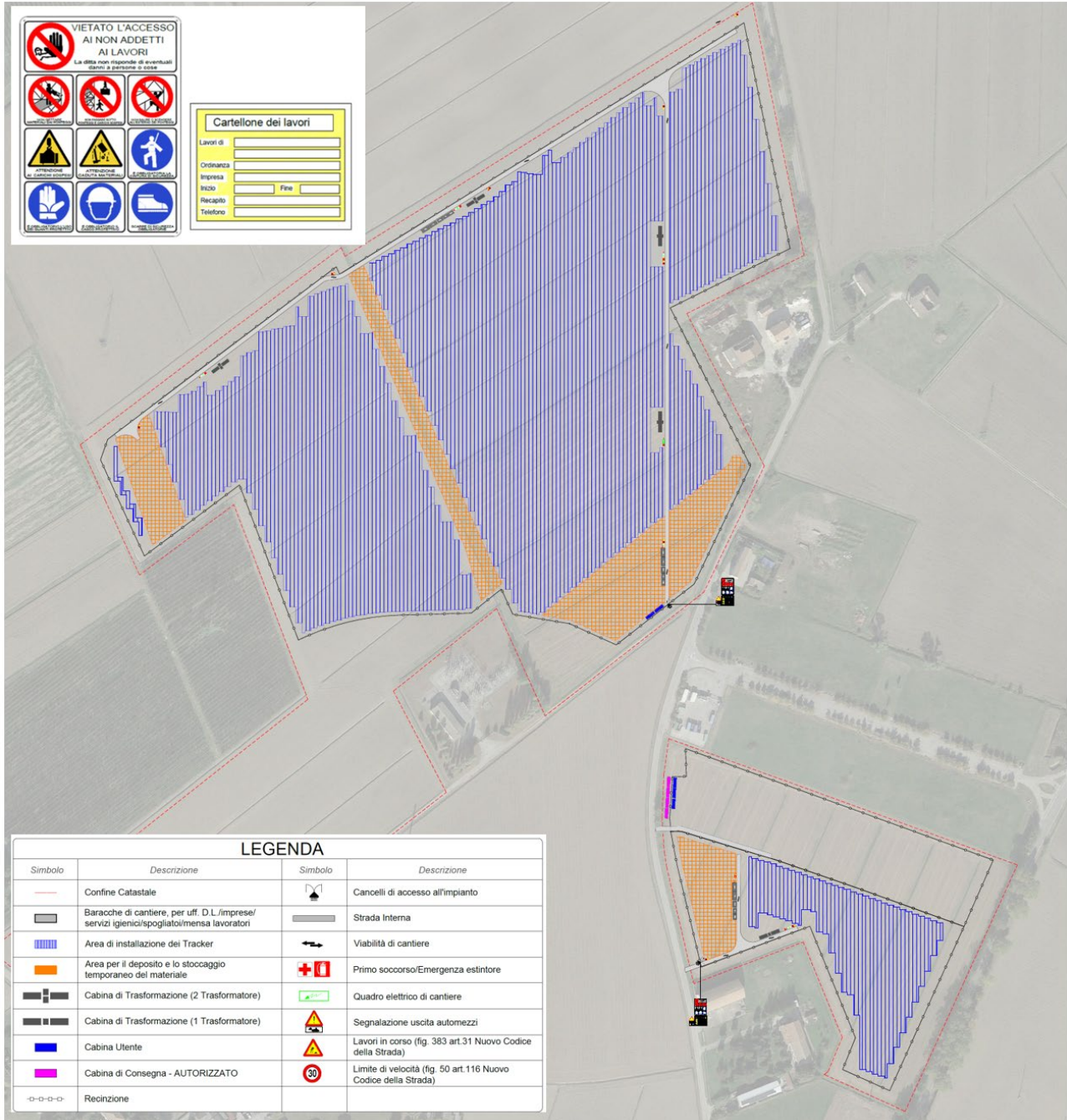
Figura 20: layout di cantiere
