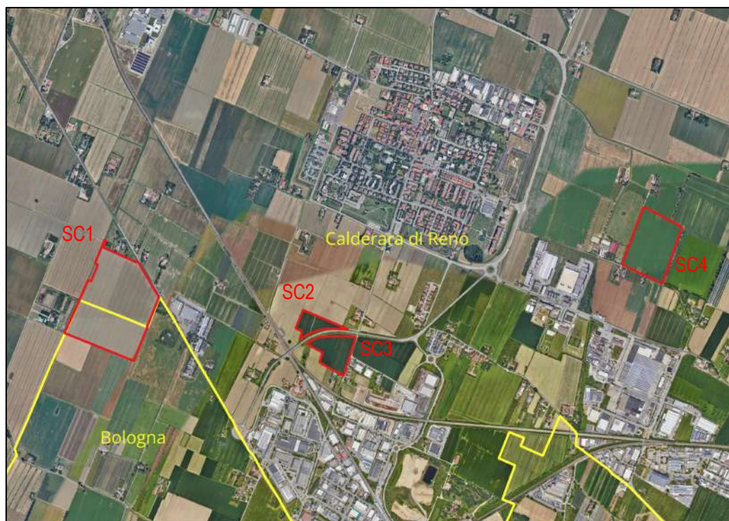
Figura 2.1: Corografia aree impianto su foto satellitare (scala 1:15.000)
