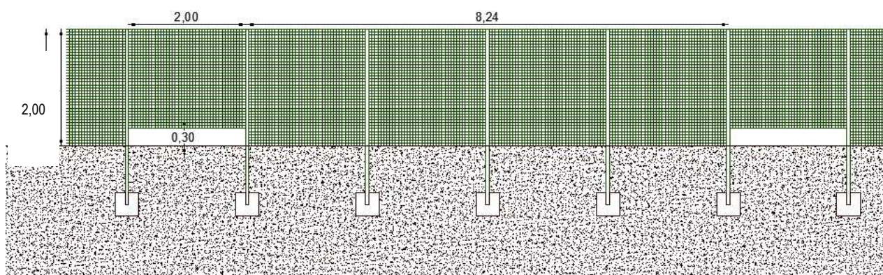
Figura 3.2: Tipologia della rete adottata
