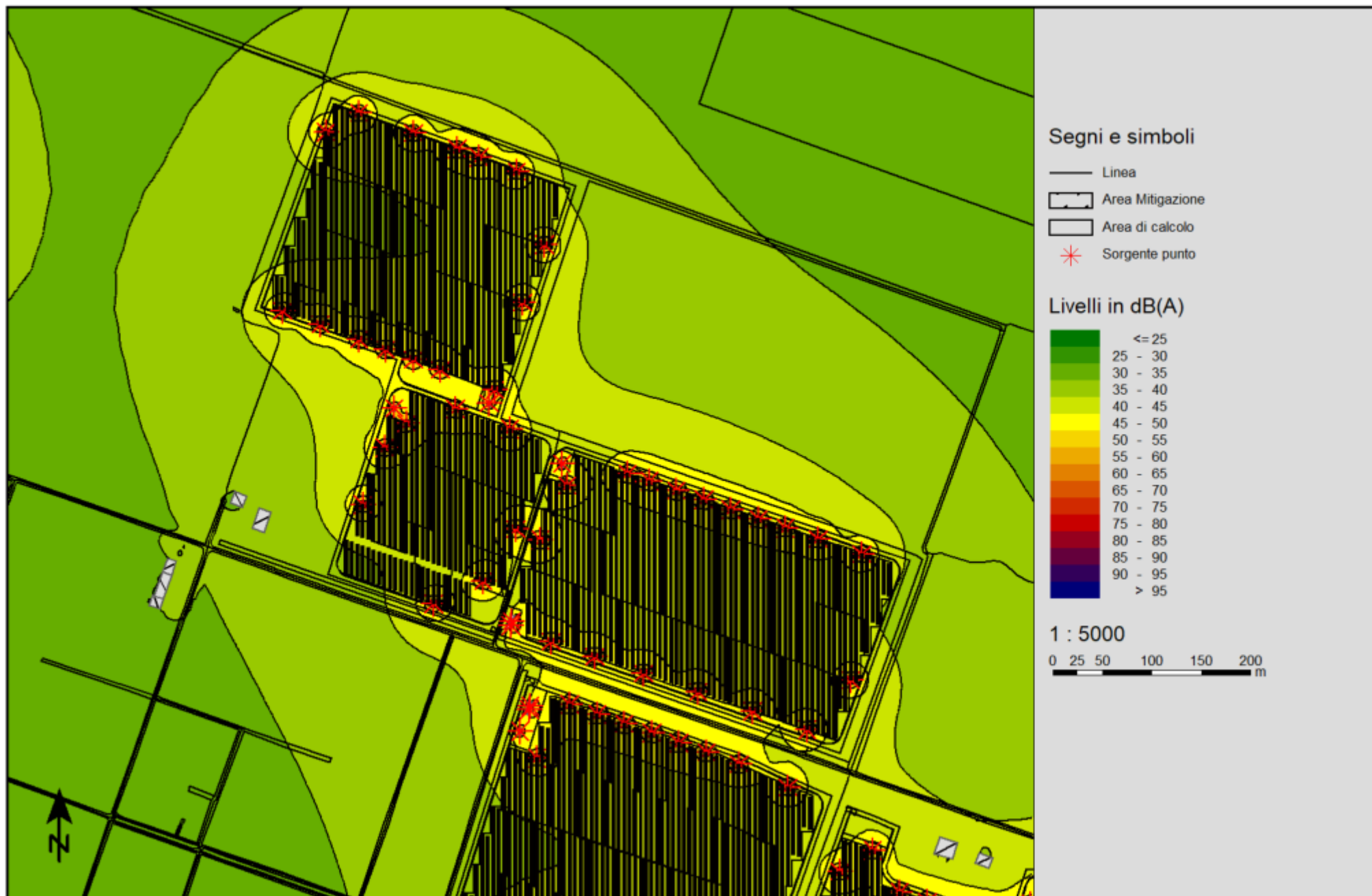
Mappa isolivello periodo diurno TR (06.00-22.00) scenario esercizio (1,5 mt) - Sorgenti fisse (emissione) – Sottocampo 2
