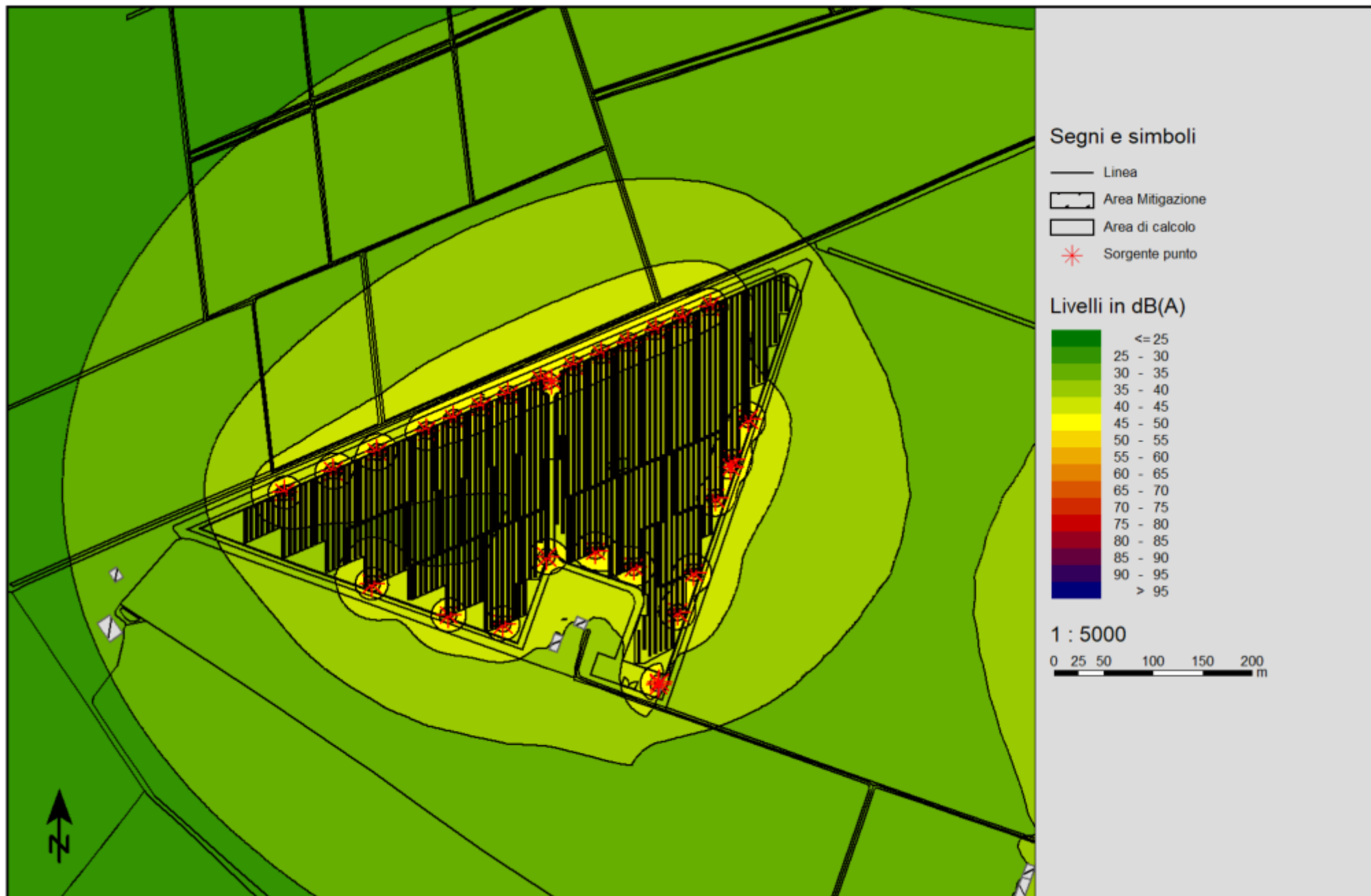
Mappa isolivello periodo diurno TR (06.00-22.00) scenario esercizio (1,5 mt) - Sorgenti fisse (emissione) – Sottocampo 1
