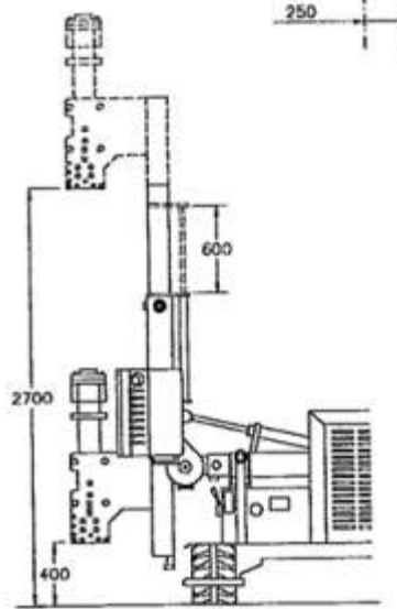
MOVIMENTAZIONE MARTELLO E COLONNA
