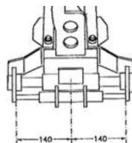
TRASLAZIONE COLONNA
