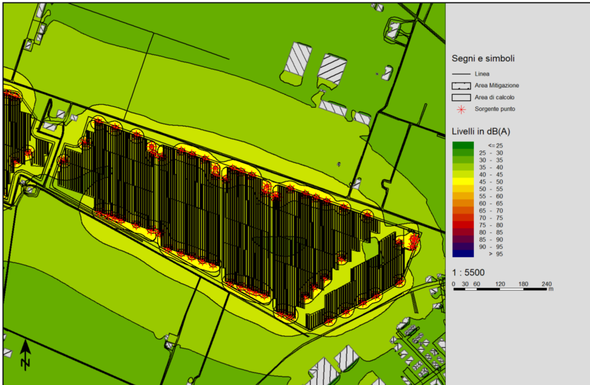
Mappa isolivello periodo diurno TR (06.00-22.00) scenario esercizio (1,5 mt) - Sorgenti fisse (emissione) – Sottocampo 3.3
