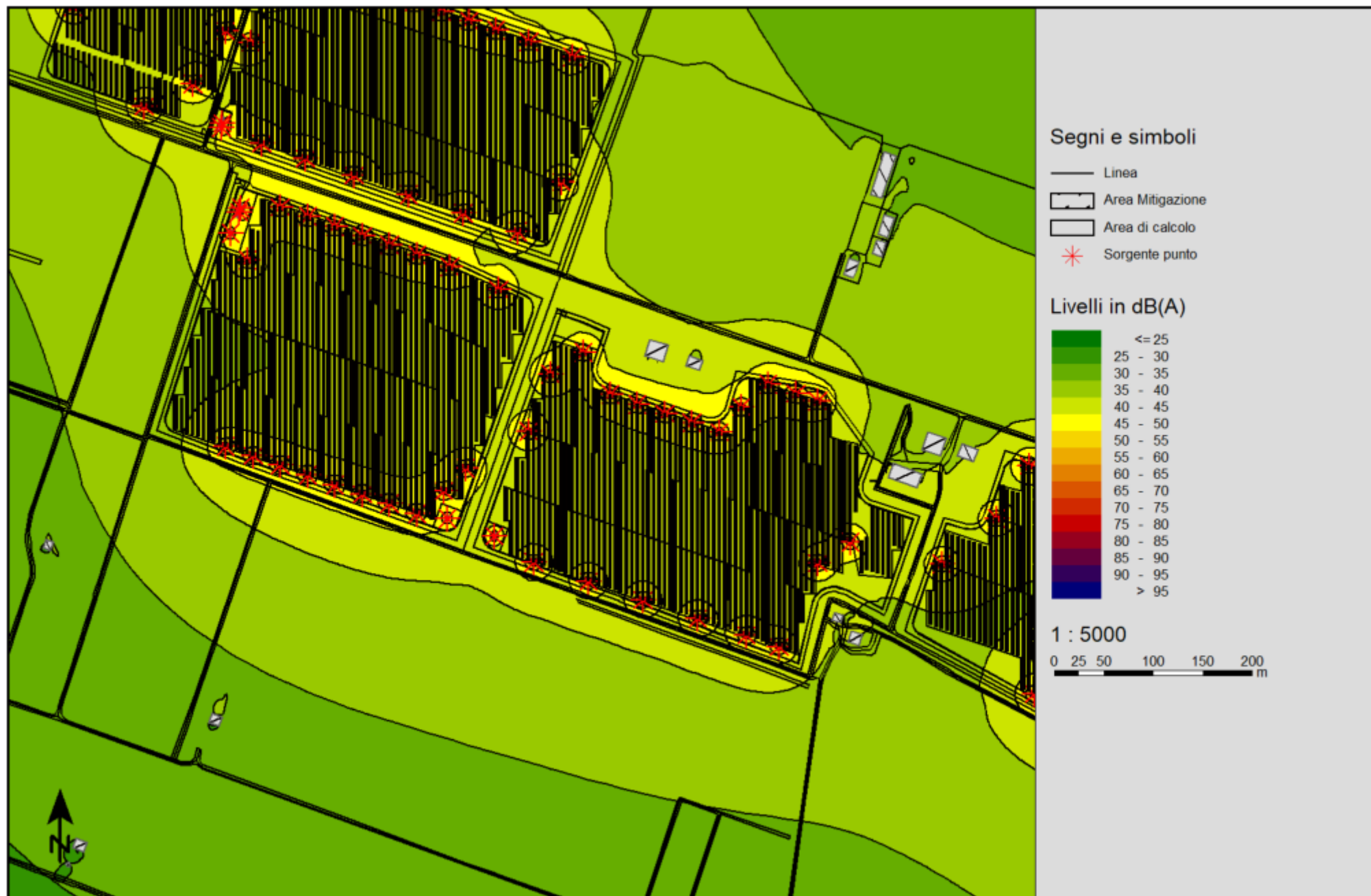
Mappa isolivello periodo diurno TR (06.00-22.00) scenario esercizio (1,5 mt) - Sorgenti fisse (emissione) – Sottocampo 3.1-3.2
