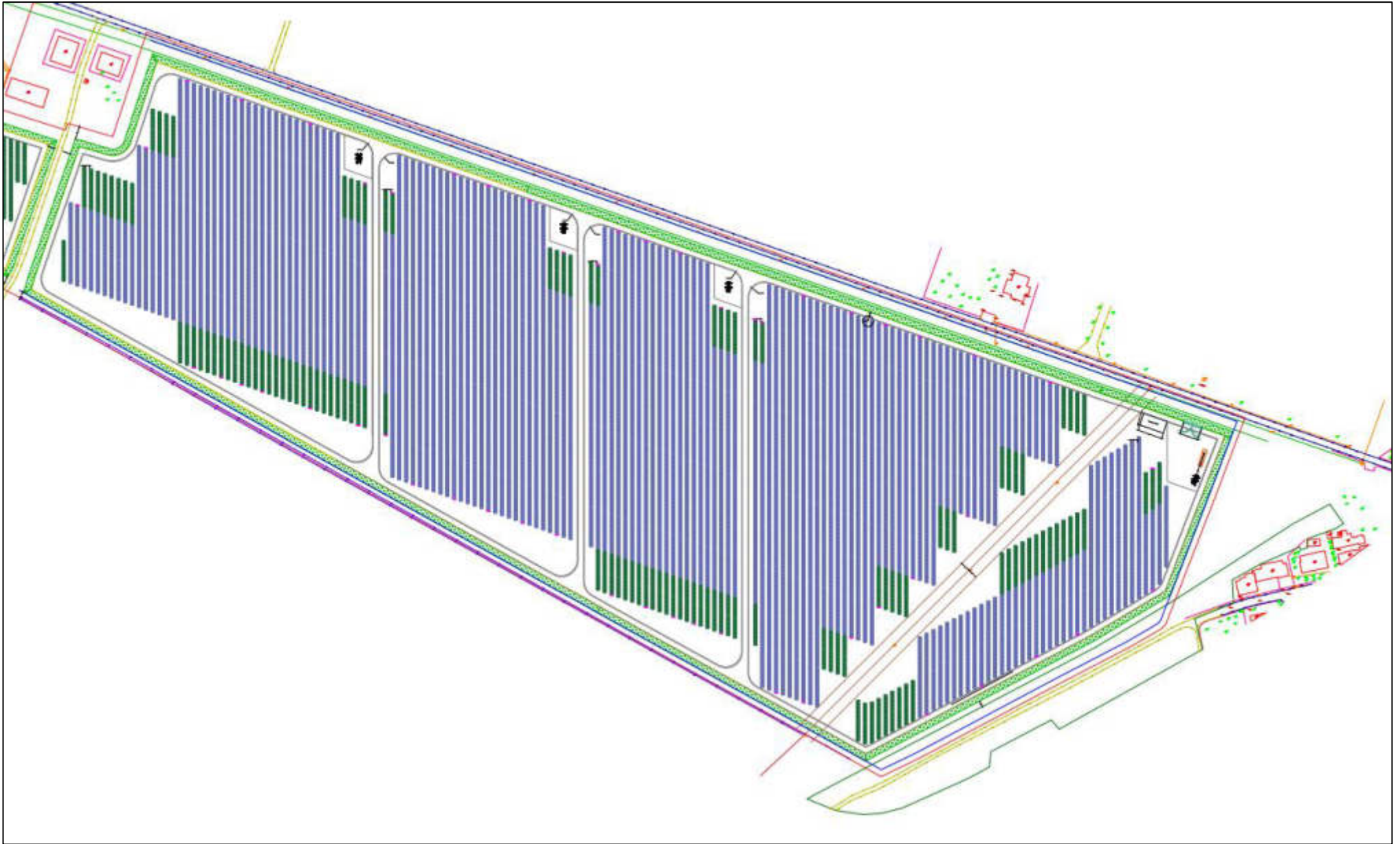
Planimetria di progetto impianto agrivoltaico – Layout sottocampo 3.3
