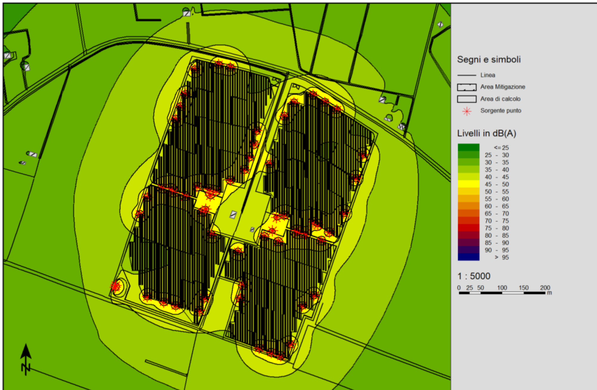
Mappa isolivello periodo diurno TR (06.00-22.00) scenario esercizio (1,5 mt) - Sorgenti fisse (emissione) – Sottocampo 4
