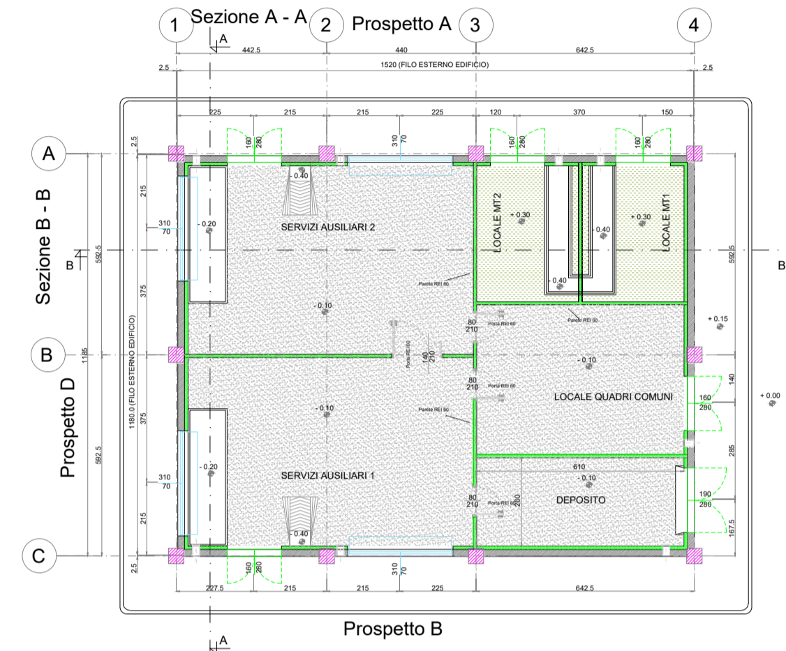
PIANTA ARCHITETTONICA
