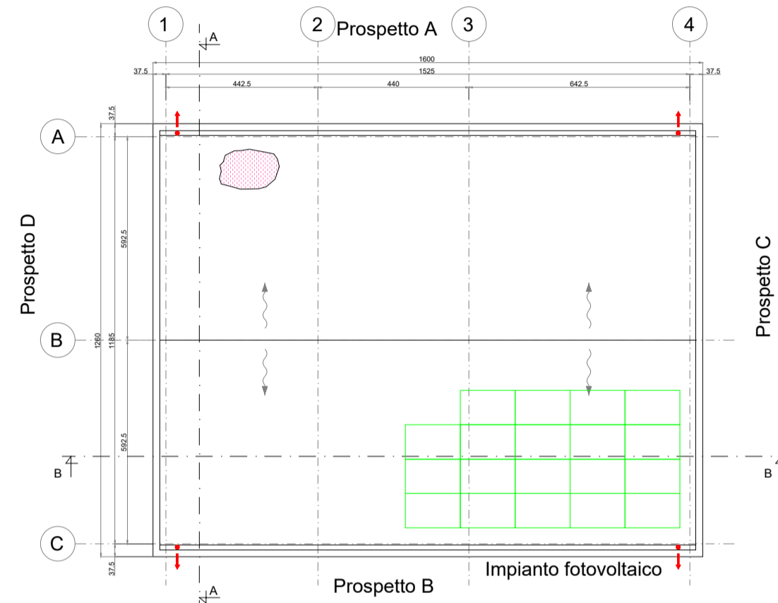
PIANTA COPERTURA
