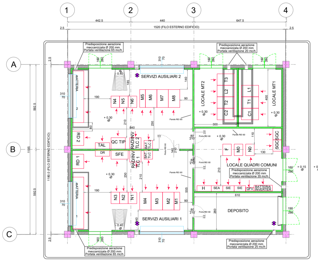
PIANTA IMPIANTISTICA
