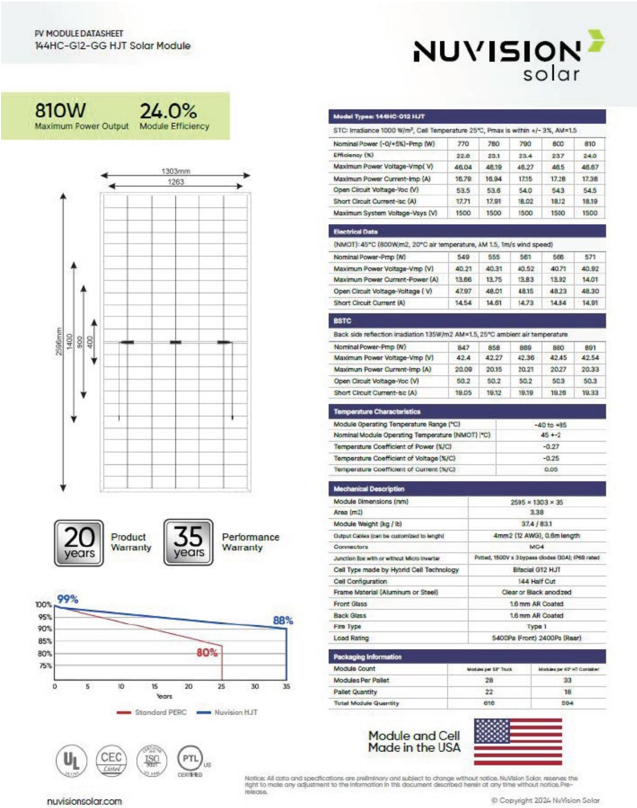
Figura 3.5: Caratteristiche Dimensionali, Elettriche e Meccaniche del Modulo
