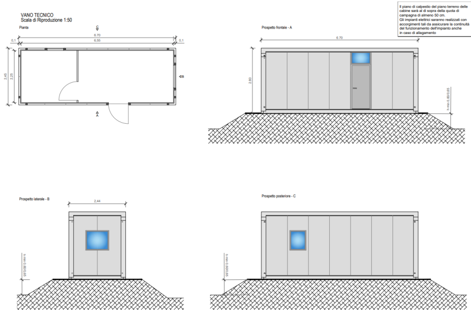
Figura 2.2: Vano Tecnico
