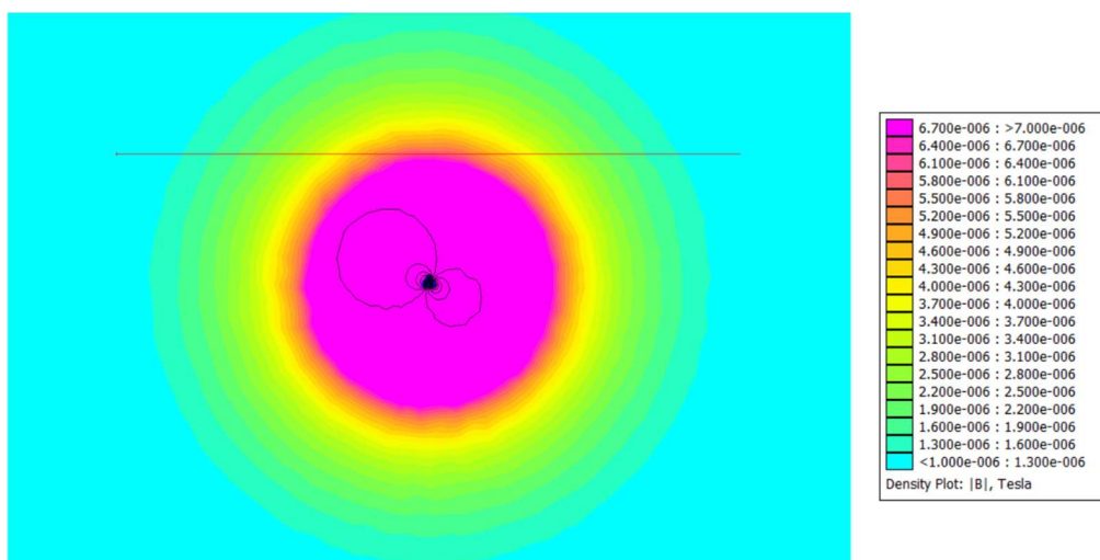
Figura 5-2: Valutazione intensità induzione magnetica tramite software FEMM. La linea rossa rappresenta il piano del suolo.
