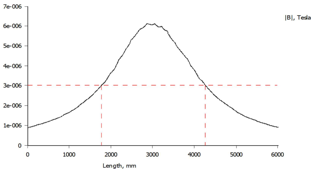
Figura 5-3: Andamento dell'intensità dell'induzione magnetica al suolo. Il cavidotto è posto in corrispondenza dell'ascissa x = 3000 \text{ mm} .
