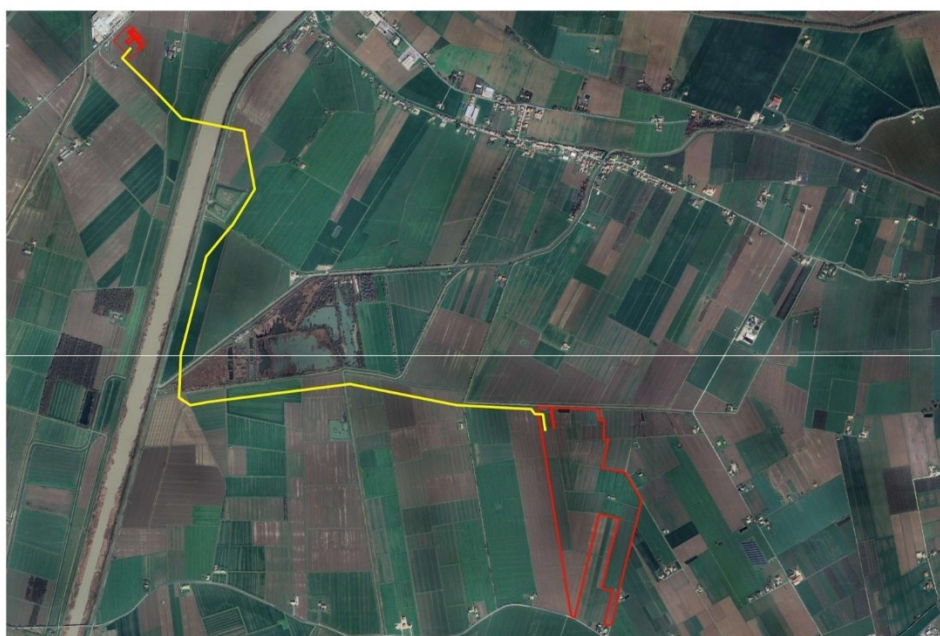
Figura 1 - Ortofoto dell'area in esame e cavidotti a 36 kV di collegamento alla nuova Stazione Elettrica della RTN
