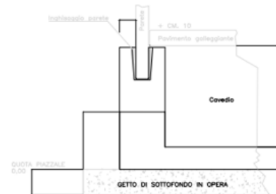
CABINA UTENTE PREFABBRICATA PARTICOLARI DI FONDAZIONE
