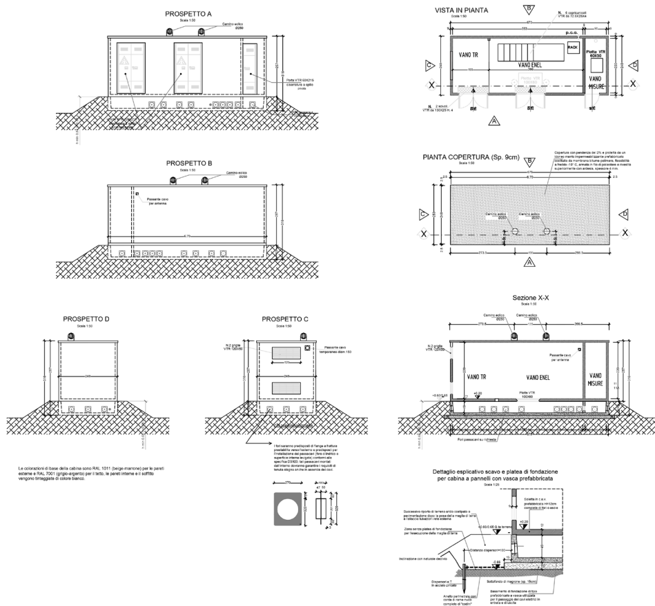
Figura 2.3: Cabina di Consegna
