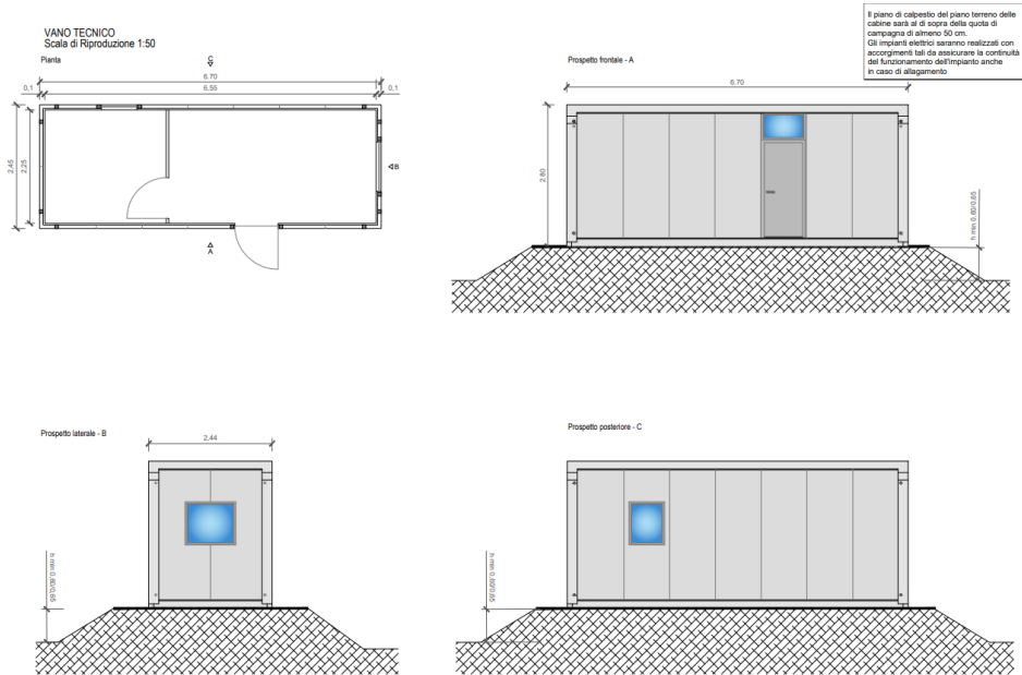
Figura 2.7: Vano Tecnico
