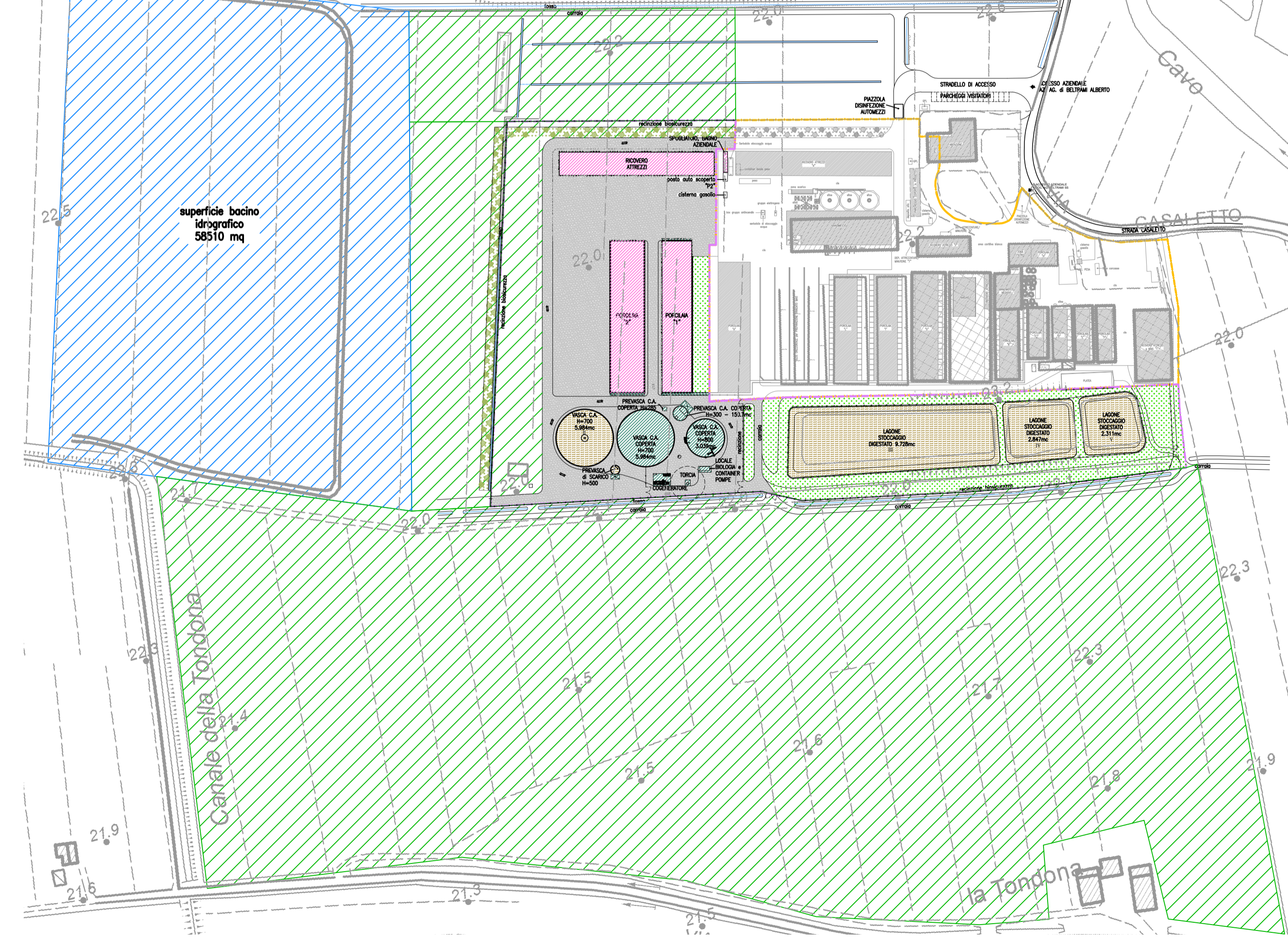
ESTRATTO C.T.R. STATO AUTORIZZATO scala 1:2000
