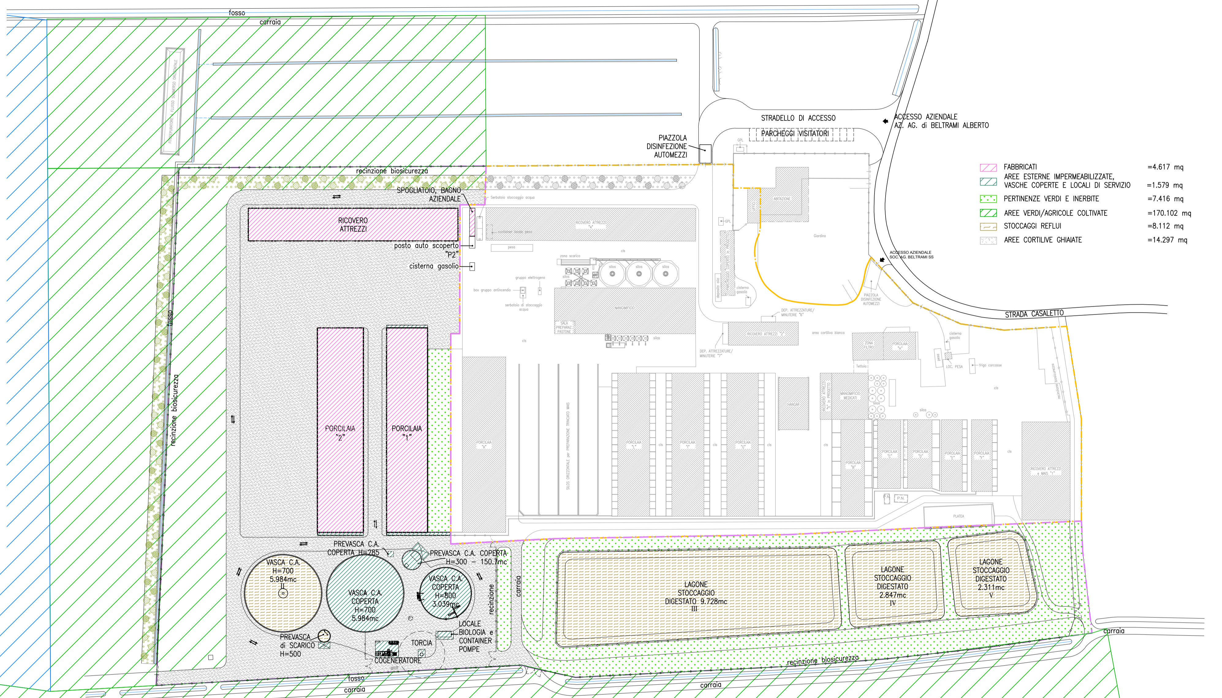
PLANIMETRIA GENERALE STATO DI PROGETTO scala 1:1000
