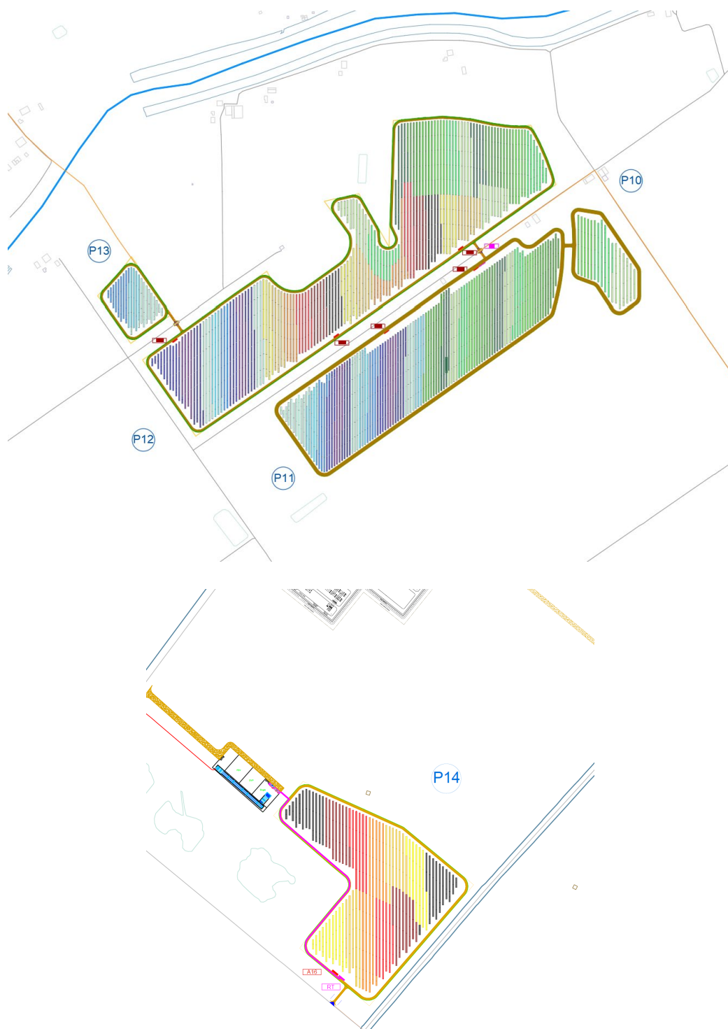
Figura 1 - Particolare schema di suddivisione sottocampi
