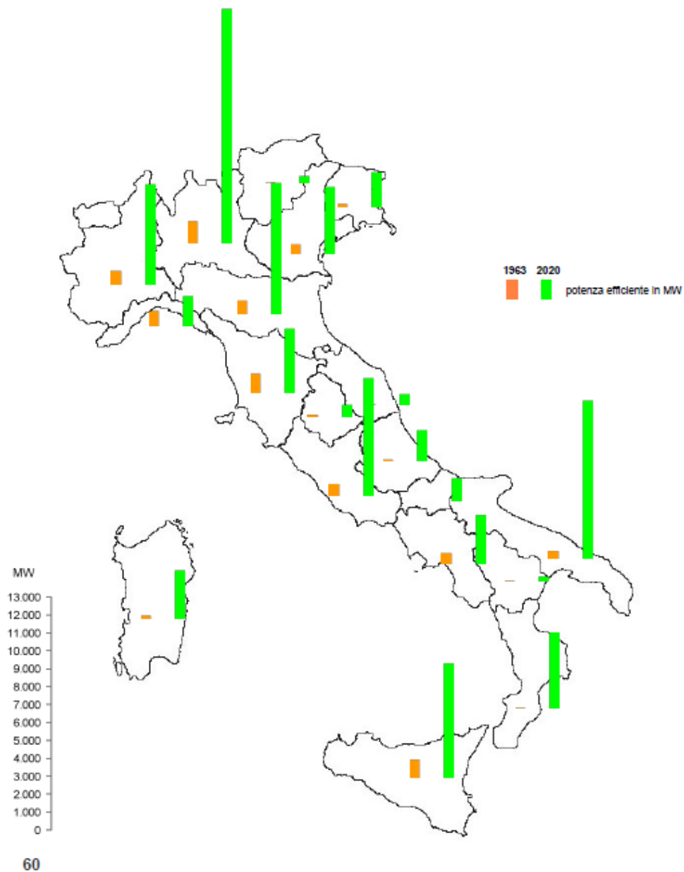
Figura 25 - Produzione termoelettrica regioni italiane
