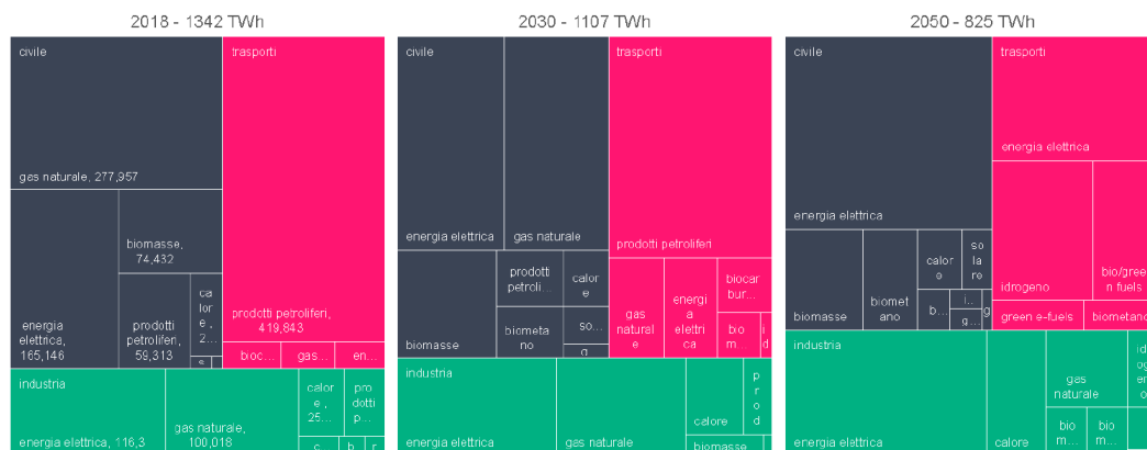
Figura 6. Consumo finale di energia anno 2018, 2030, 2050 simulazione RSE.
