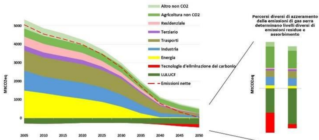
Figura 5 - emissioni gas serra in scenario 1,5°
