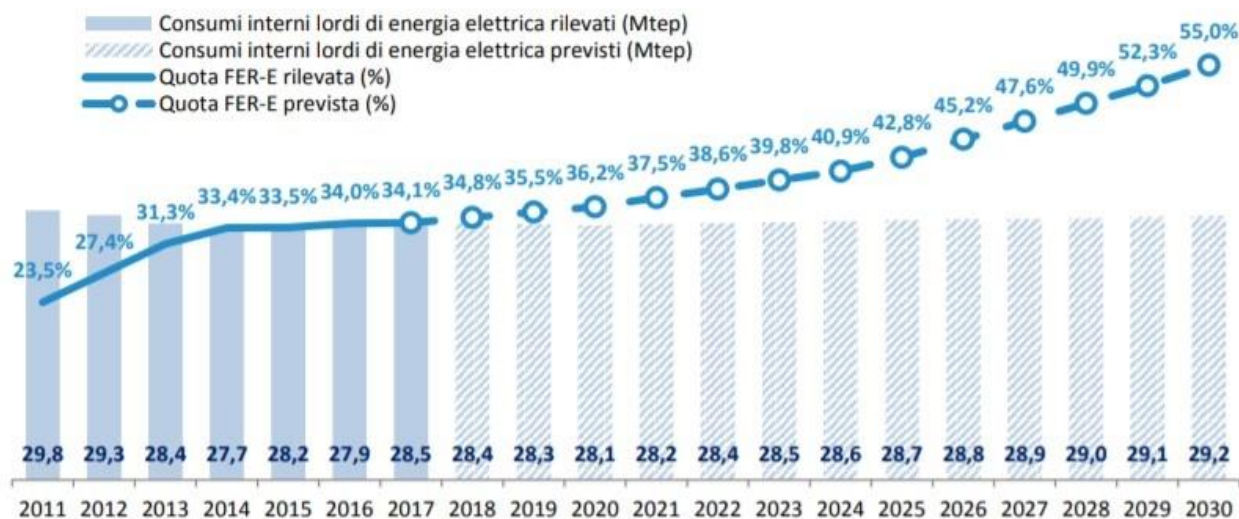
Figura 33 - Percorso FER elettriche
