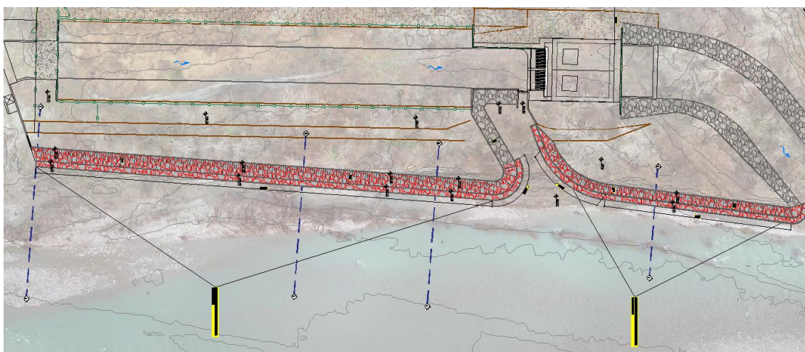
Figura 12 - stralcio planimetrico con l'indicazione delle due difese spondali previste
