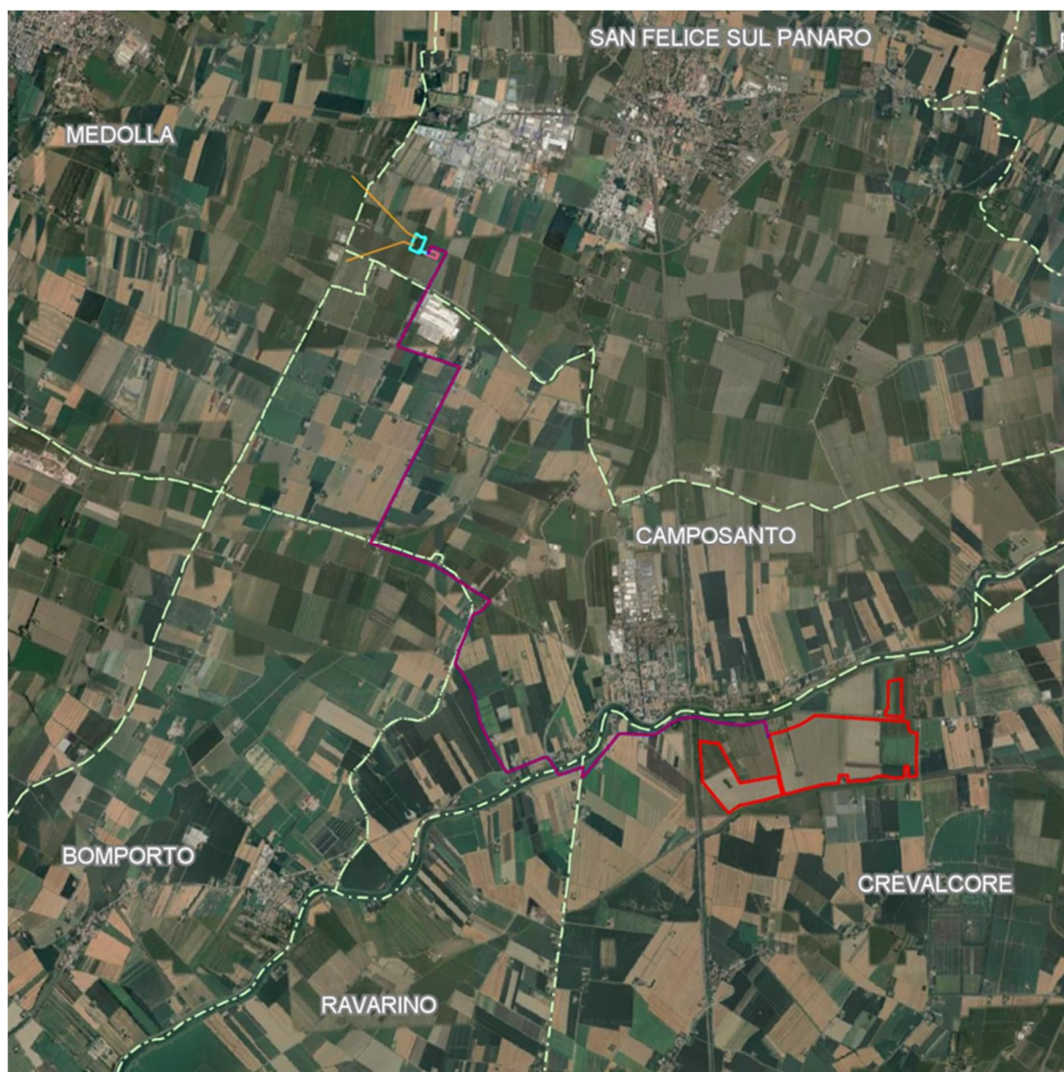
Figura 1 - Inquadramento su base ortofoto delle opere in progetto con evidenza dei confini Comunali. In rosso il perimetro di impianto, in viola il cavidotto AT, separata a Nord in magenta la SEU Condivisa con altri operatori ed in ciano la Stazione di Terna, in oro sono rappresentate le connessioni aeree
