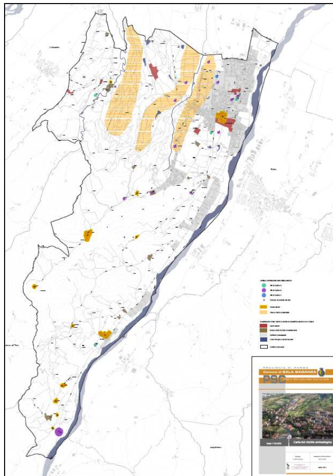
Figura 7 – PSC 2011 di Sala Baganza, Carta del rischio archeologico
