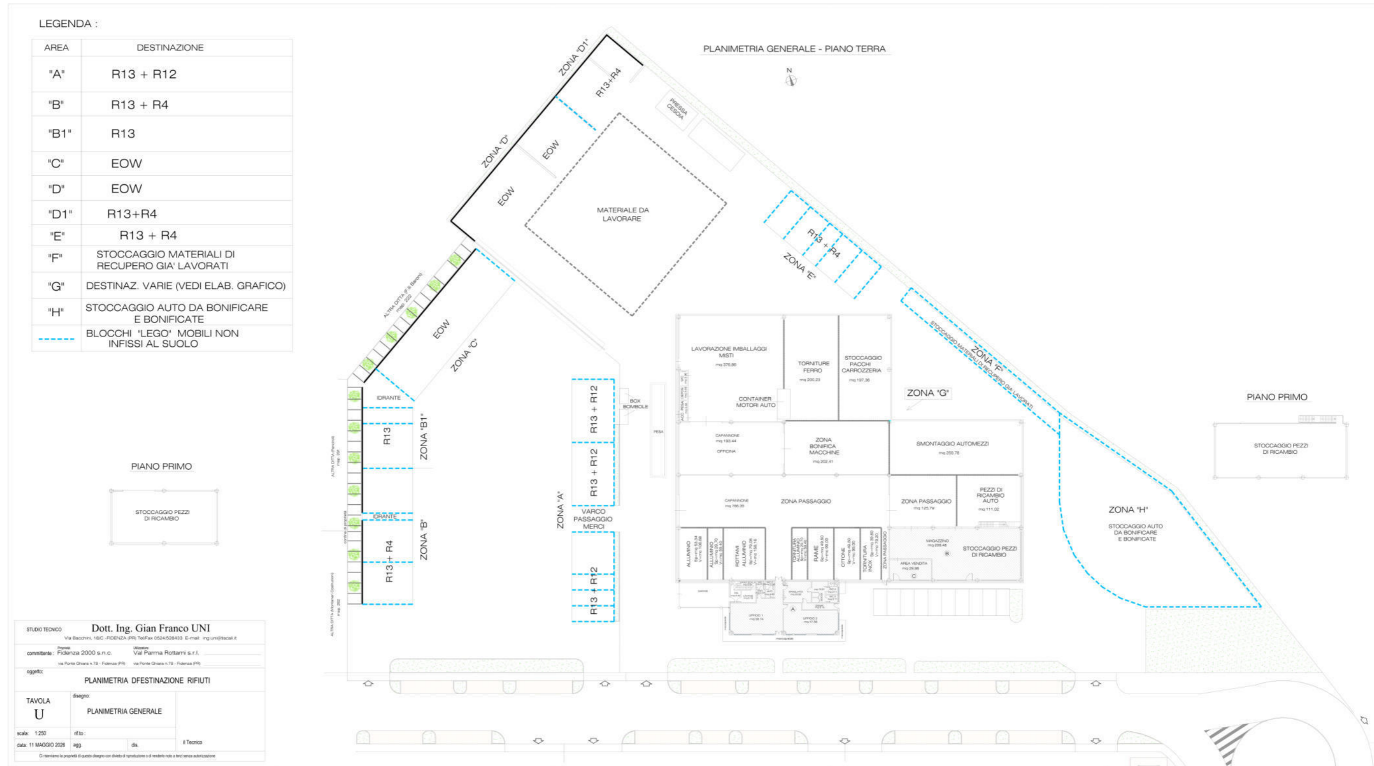
Figura 5 – Tavola U – Planimetria destinazione rifiuti (fuori scala).
