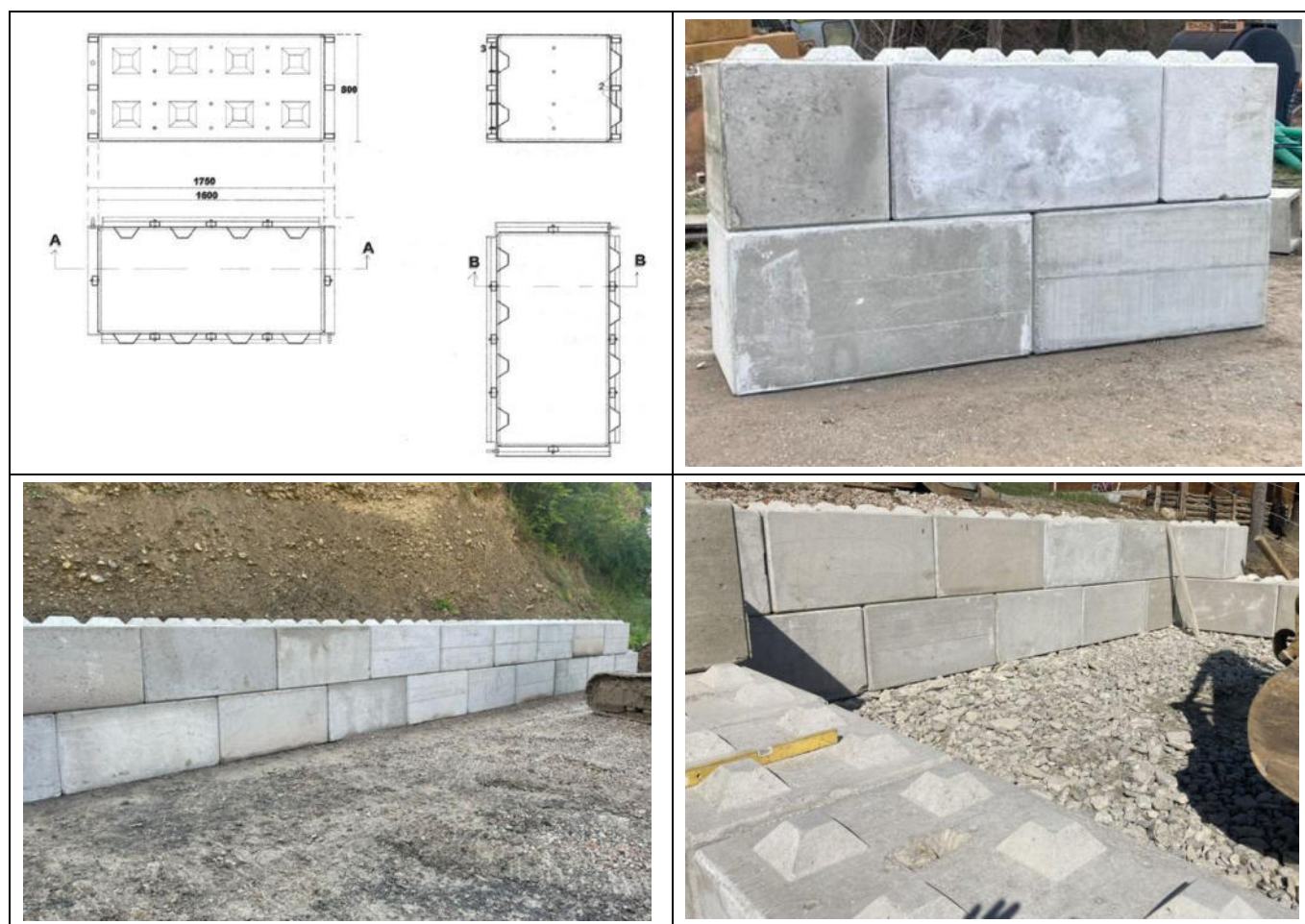
Figura 6 – Immagini esemplificative delle barriere mobili del sistema Block Art®, di delimitazione dei box/baie per la messa in riserva/trattamento dei rifiuti e per lo stoccaggio EoW.
