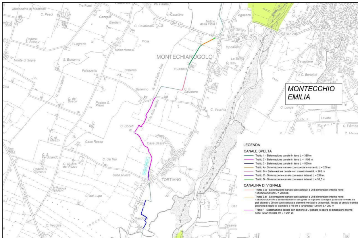
FIG. 2.1 – PLANIMETRIA DI PROGETTO LOTTO II TRATTO CANALE SPELTA.
