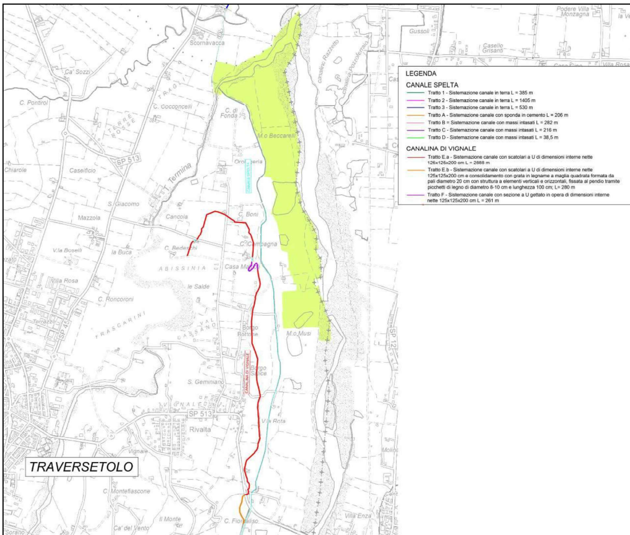
FIG. 2.2 – PLANIMETRIA DI PROGETTO LOTTO II TRATTO CANALE VIGNALE.
