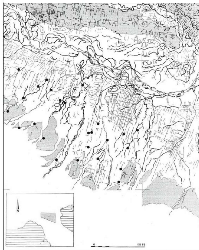
FIG. 6.1 CARTA DEI PALEOALVEI E LOCALIZZAZIONE DELLE TERRAMARE EMILIANE (MUTTI 1993).
