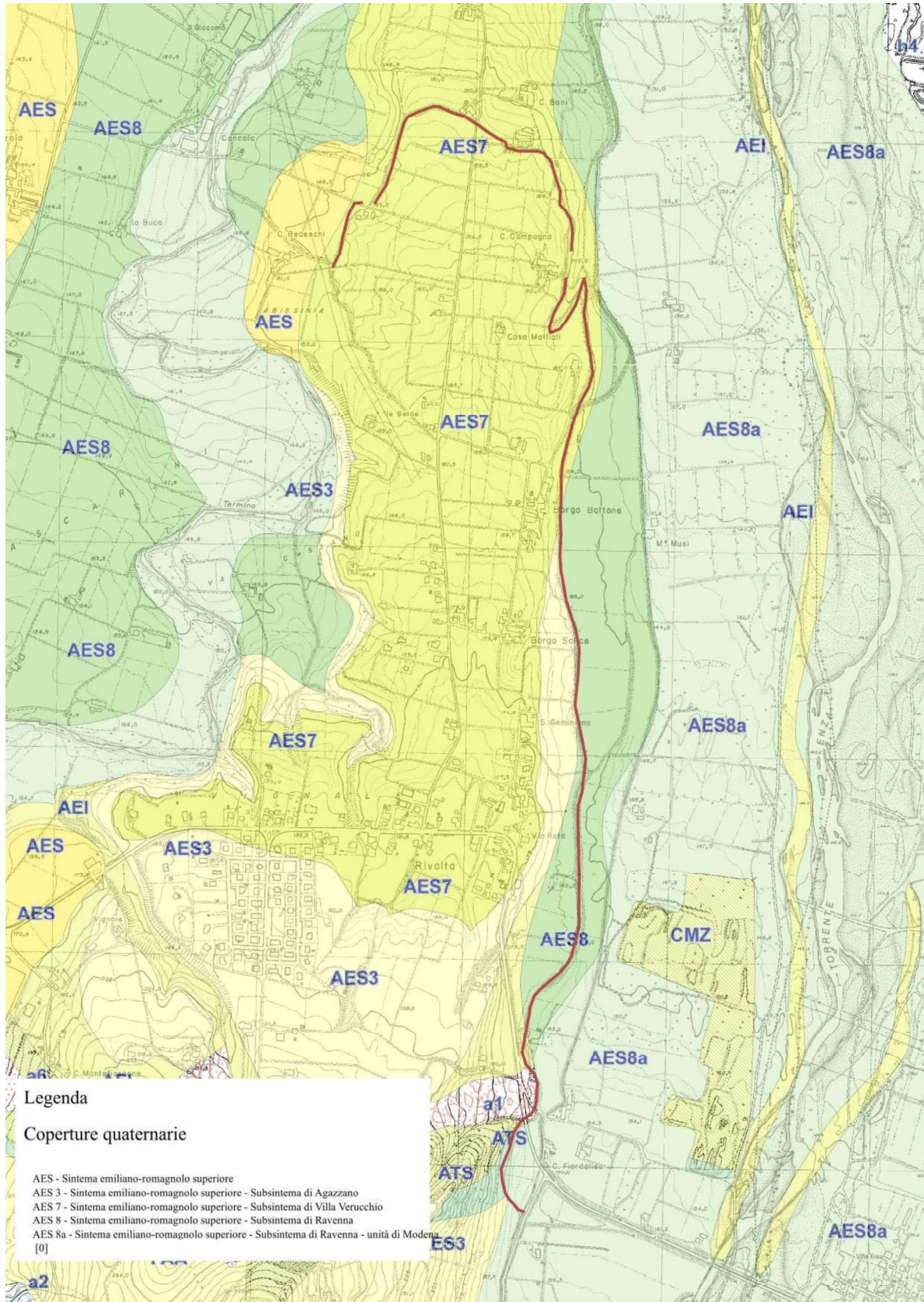
Fig. 5.2 – Tavola con le coperture quaternarie presente nell'area oggetto di intervento.
