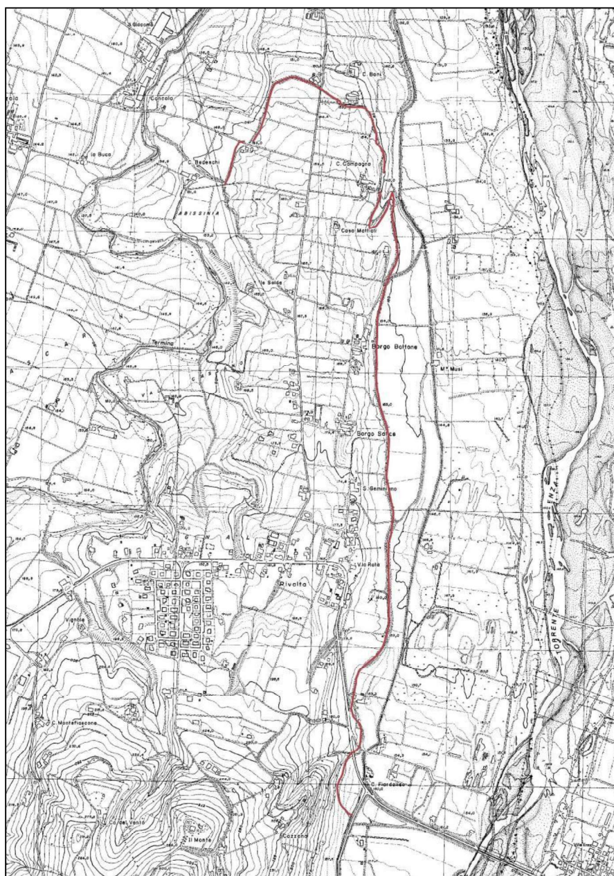
FIG. 5.1 INQUADRAMENTO DEL CANALE SPELTA E DELLA CANALINA VIGNALE SU CTR.
