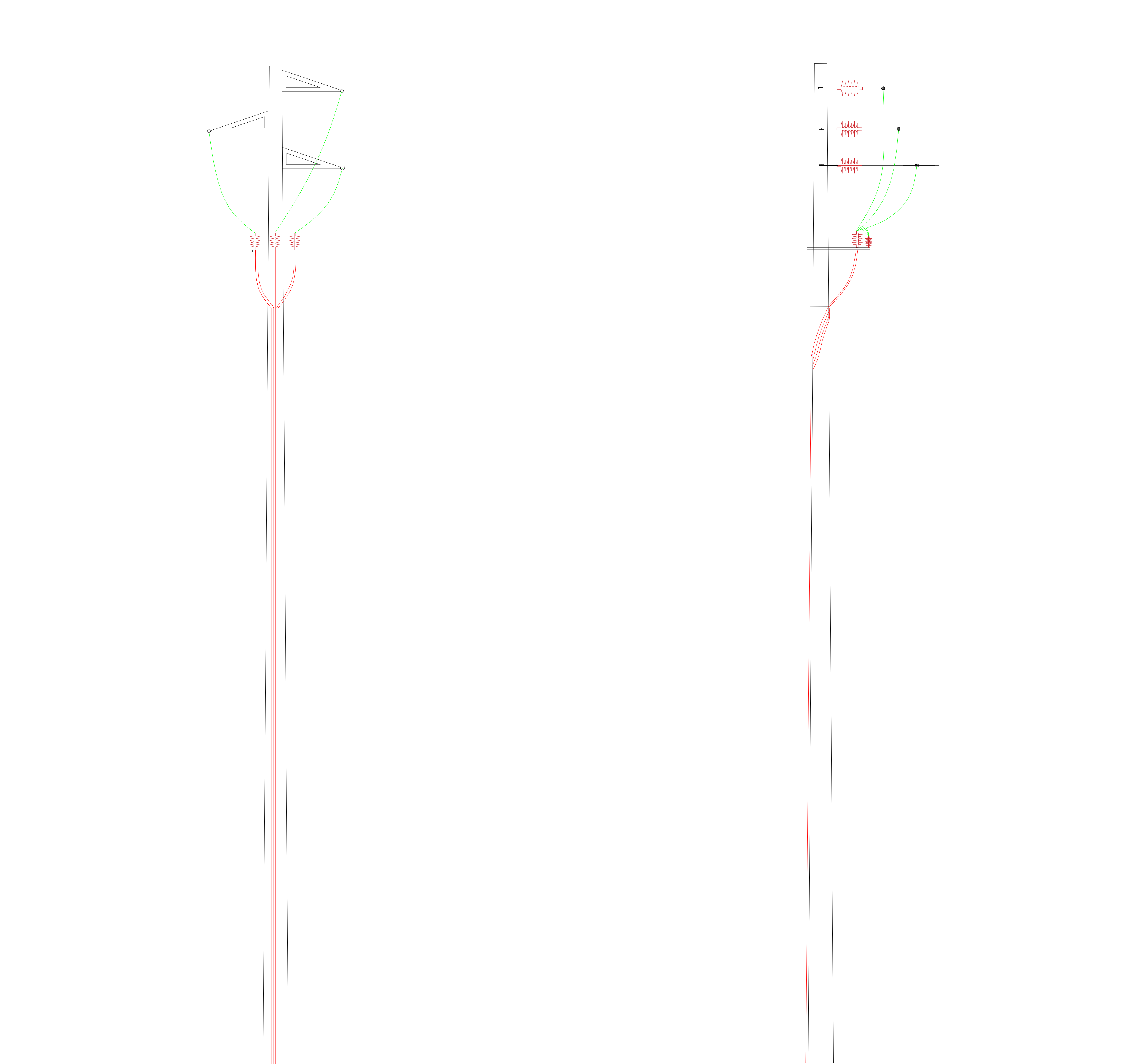
Vista frontale e laterale nuovo sostegno (da linea MT aerea a linea MT interrata)
