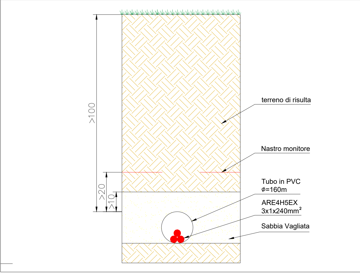
Sezione nuova linea MT Interrata
