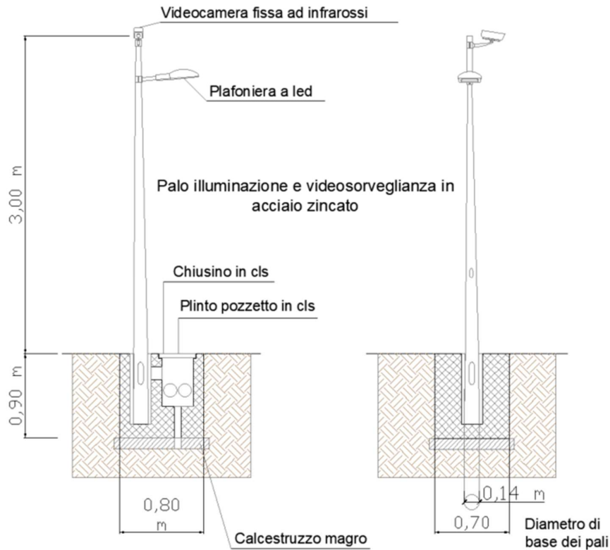
Figura 12 - Rappresentazione pali per illuminazione e videosorveglianza
