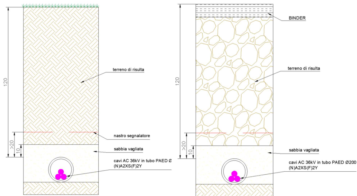
Figura 7 – Sezione tipo Opere Utente
