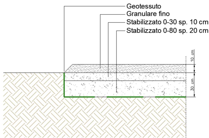
Figura 10 - Sezione tipo viabilità interna all'impianto e piazzali
