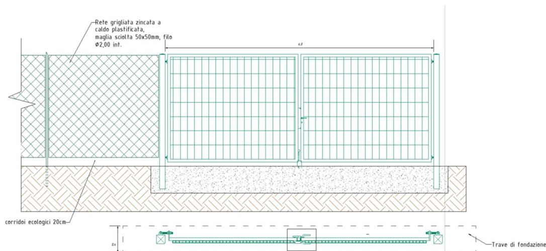
Figura 11 - Rappresentazione della recinzione prevista di altezza pari a 2.5m
