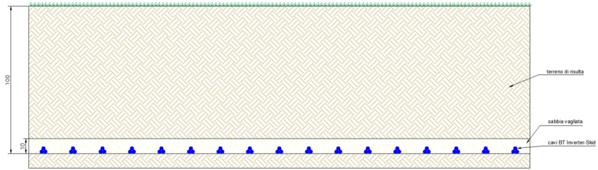
Figura 5 - Sezioni tipo inverter - Skid
