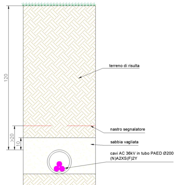
Figura 6 - Sezione tipo 36 kV skid – cabina raccolta
