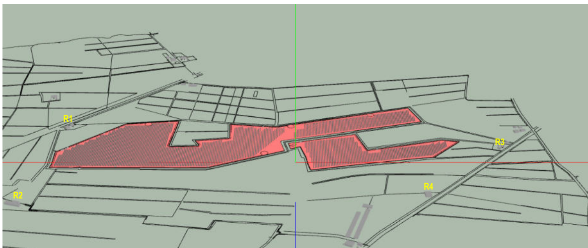
Mapa ambiente propagazione (modello previsionale) con indicazione area campo fotovoltaico e ricettori individuati
