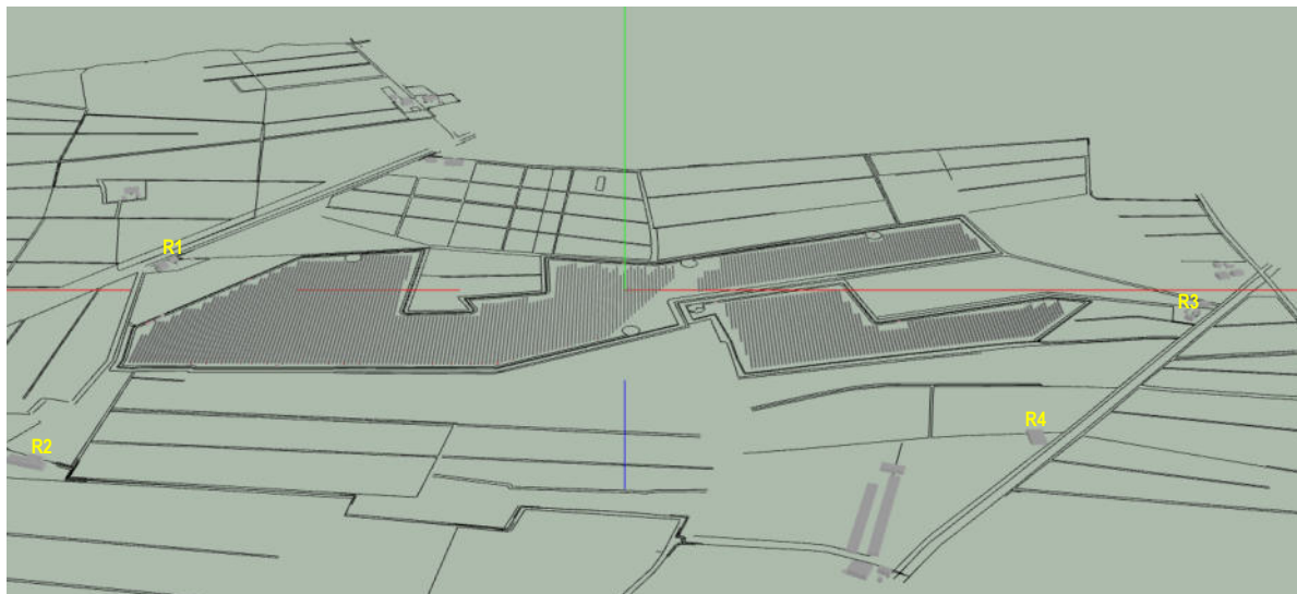
Mapa ambiente propagazione (modello previsionale) con indicazione area campo fotovoltaico e ricettori individuati
