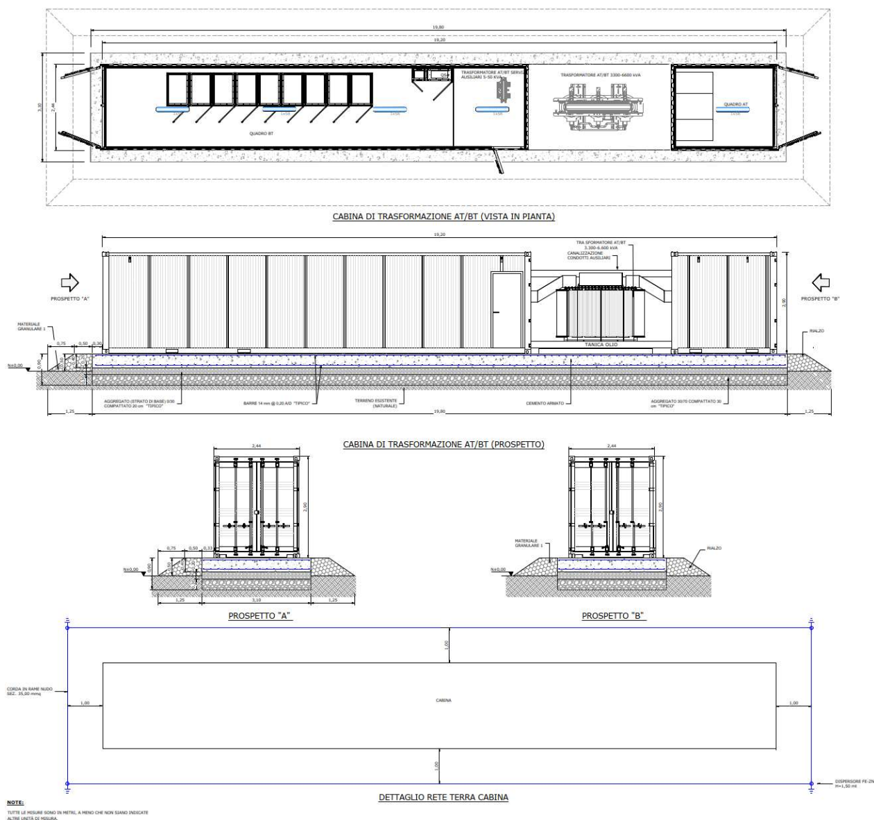
Figura 14 - Cabina di trasformazione AT/BT
