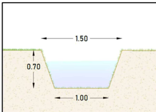
Figura 17 – Sezione tipo canali di progetto interni ai lotti
