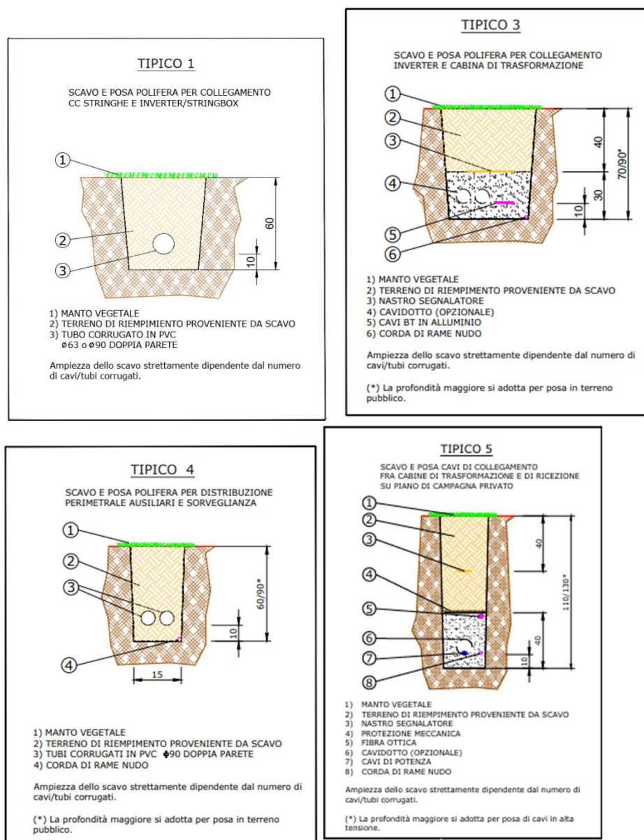
Figura 13 - Tipici scavi e posa cavi
