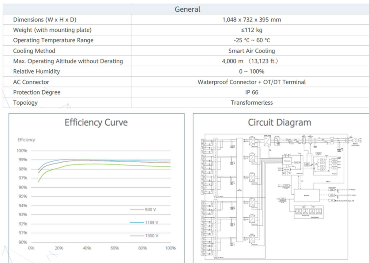
Figura 8 - Dimensioni, specifiche tecniche e prestazionali dell'inverter
