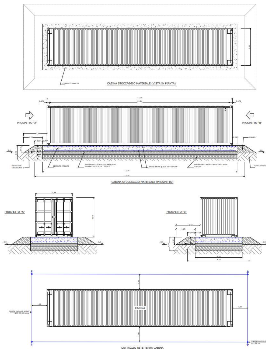
Figura 16 - Cabina di stoccaggio materiale
