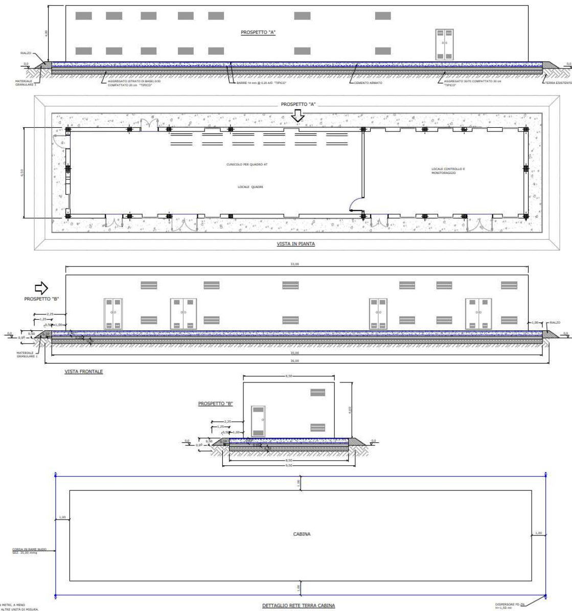
Figura 15 - Cabina di ricezione, sezionamento e controllo
