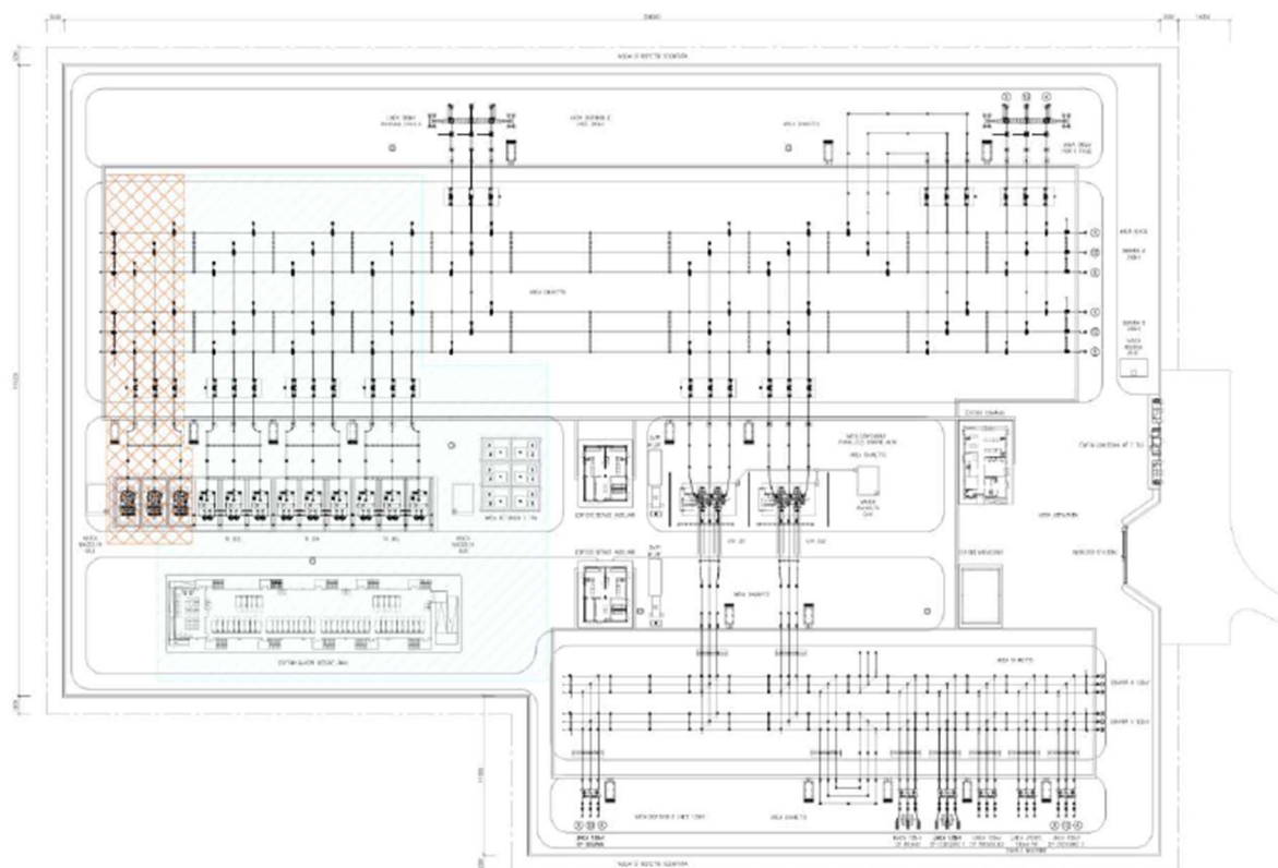
Figura 20- Planimetria elettromeccanica SE 380/132/36 kV "Fiscaglia"
