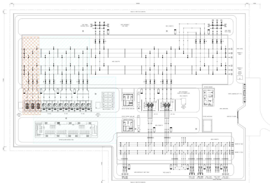
Figura 4 - Planimetria elettromeccanica SE 380/132/36 kV "Fiscaglia"
