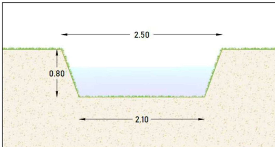
Figura 18 – Sezione tipo canali perimetrali di progetto
