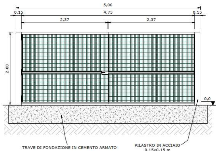
Figura 11 - Cannello a doppia anta
