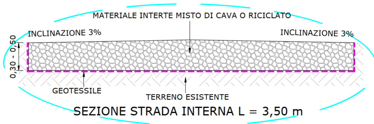
Figura 13 - Viabilità interna
