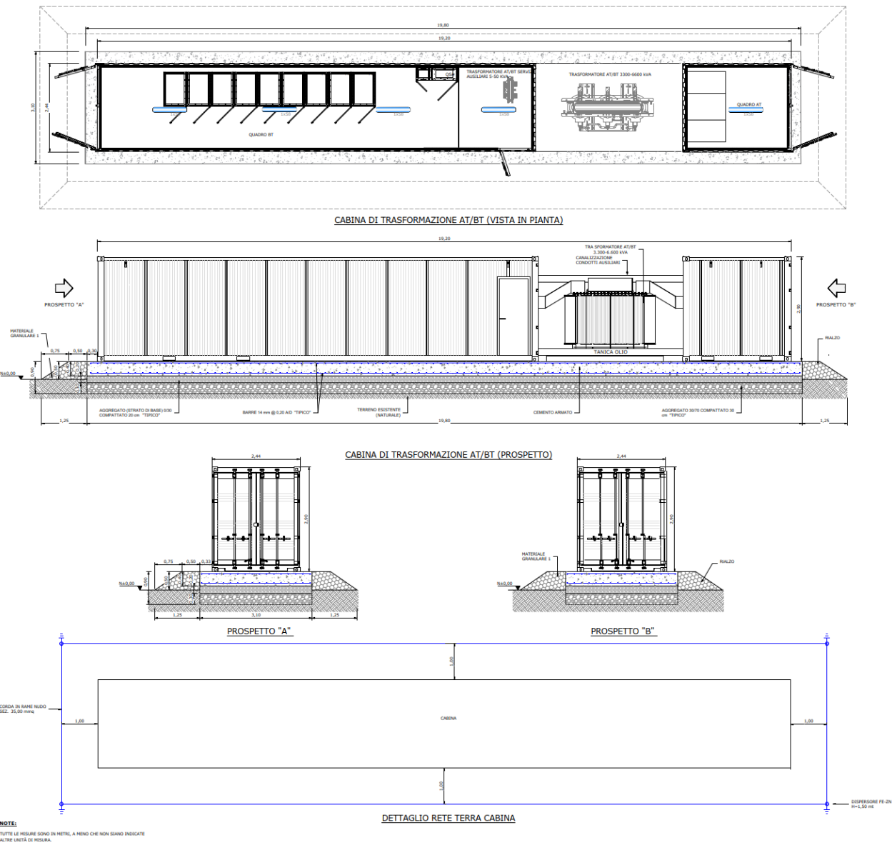
Figura 15 - Cabina di trasformazione AT/BT
