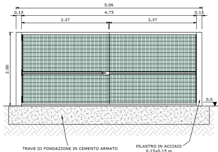
Figura 12 - Cannello a doppia anta
