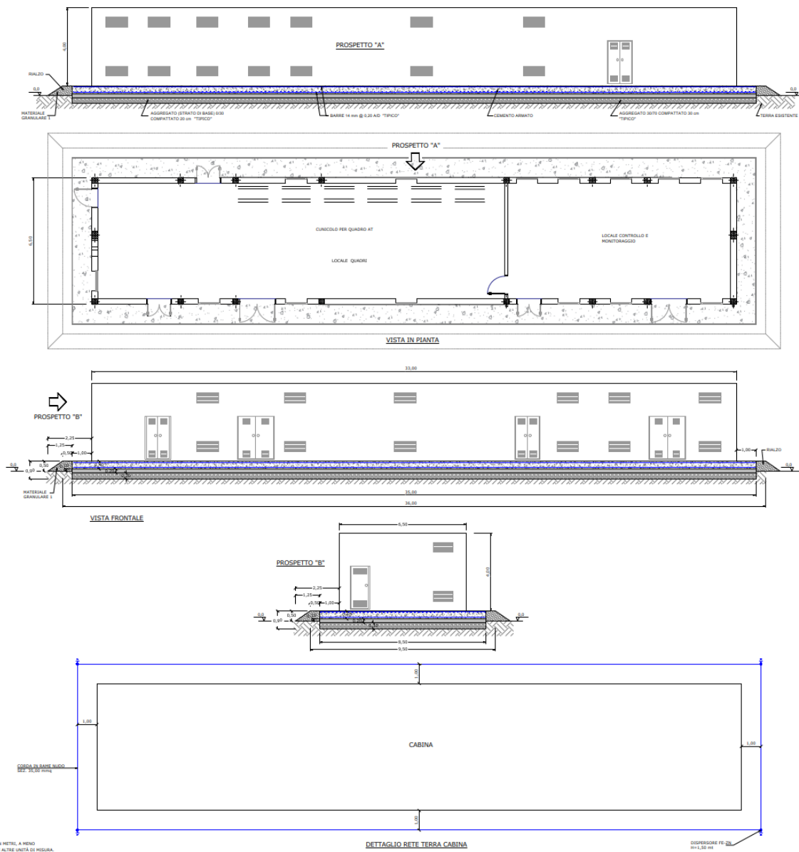
Figura 16 - Cabina di ricezione, sezionamento e controllo
