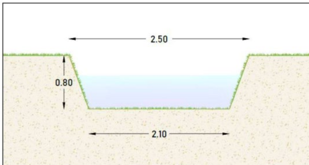
Figura 19 – Sezione tipo canali perimetrali di progetto
