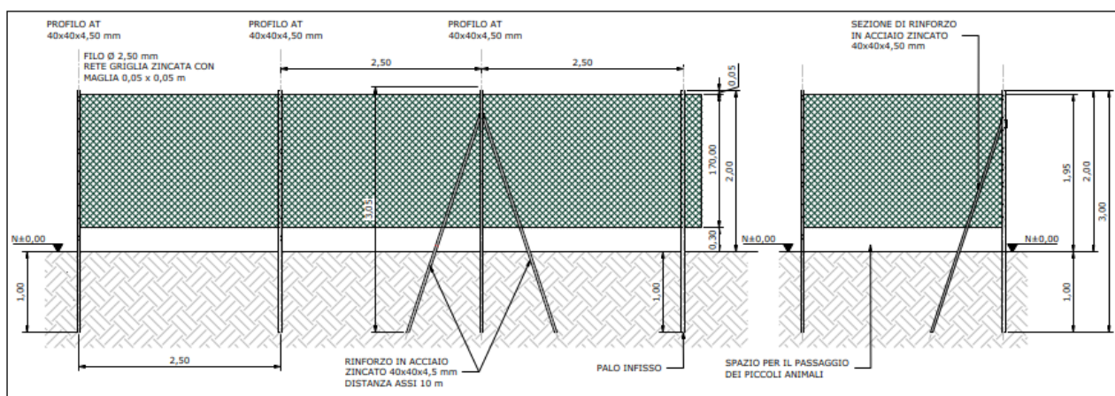
Figura 11 - Recinzione perimetrale
