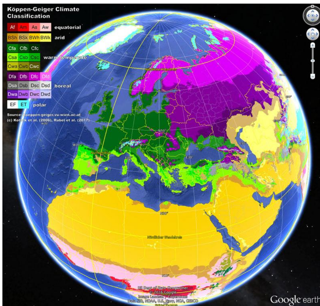
Figura 11. Inquadramento climatico globale secondo la classificazione di Koppen-Geiger. (fonte: https://koeppen-geiger.vu ).
