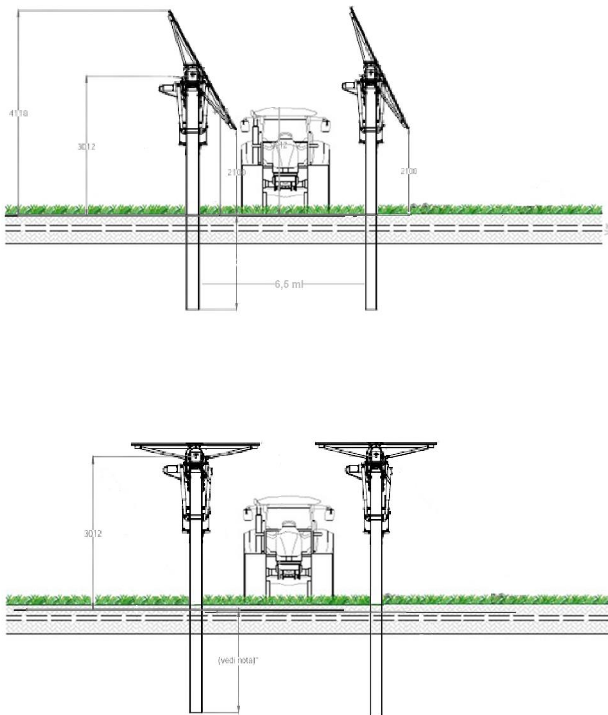
Figura 27 - Compatibilità macchinari impianto
