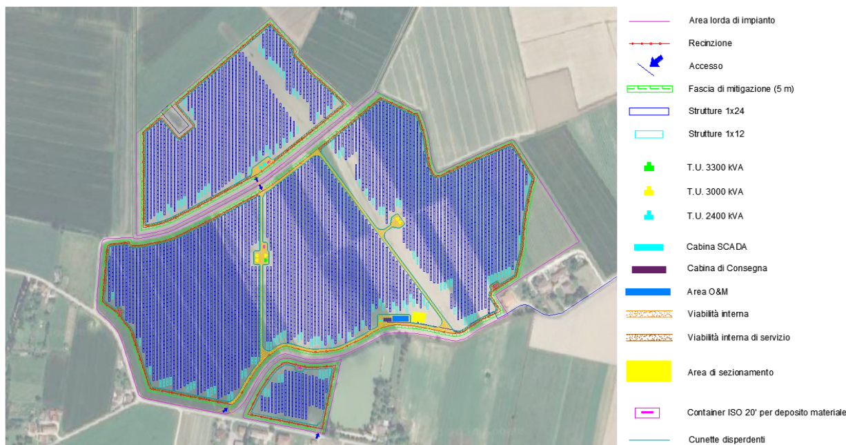
Figura 28 - Inquadramento su base ortofoto del layout di impianto
