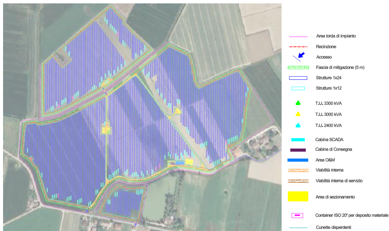
Figura 1. Layout di impianto con relative caratteristiche
