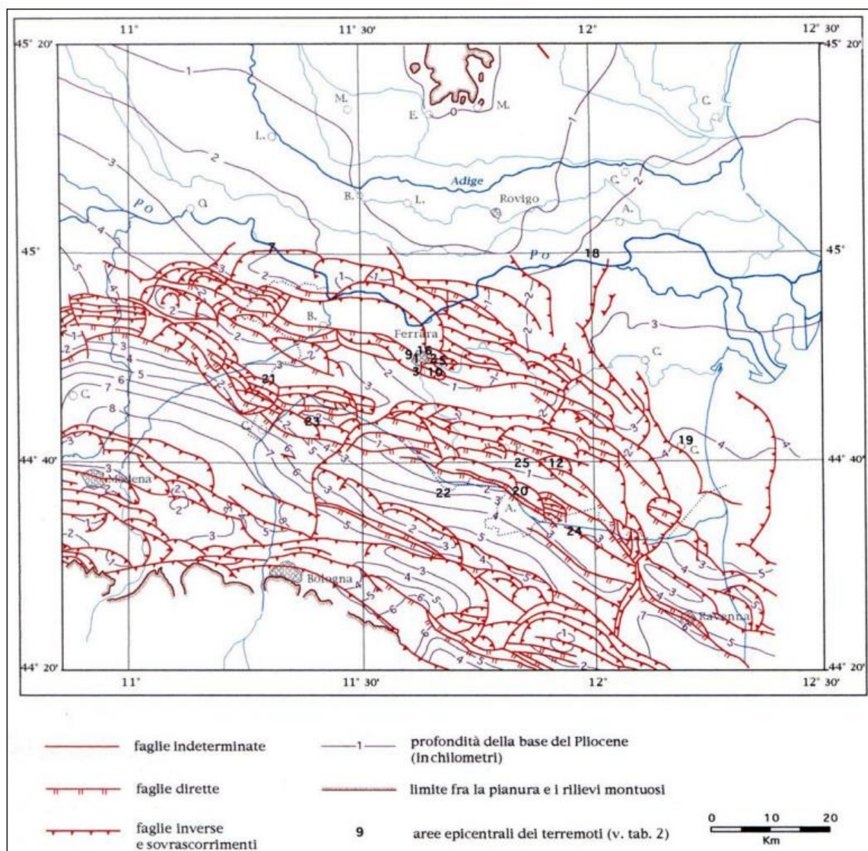
Figura 6 - Carta strutturale della Pianura Padana orientale (Pieri e Groppi, 1981, CNR, 1992)
