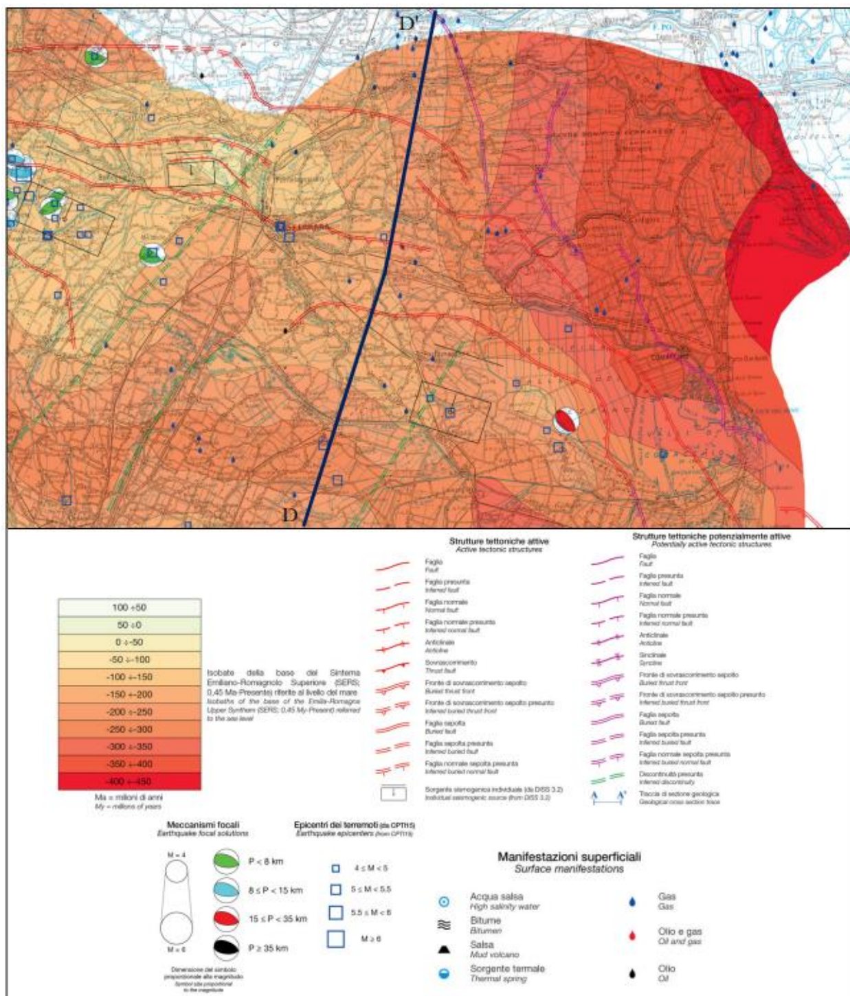
Figura 10 - Stralcio centrato sul comune di Voghiera della nuova carta sismotettonica dell'Emilia Romagna (anno 2017). (Carta sismotettonica della Regione Emilia Romagna - 2016).
