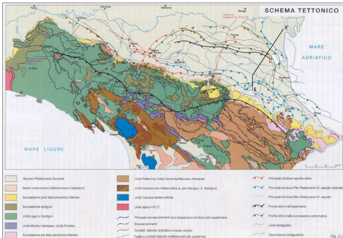
Figura 7 – “Schema Tettonico”, tratto da “Carta Sismotettonica della Regione Emilia-Romagna” a cura di Luca Martelli e Mario Boccaletti (2004)
