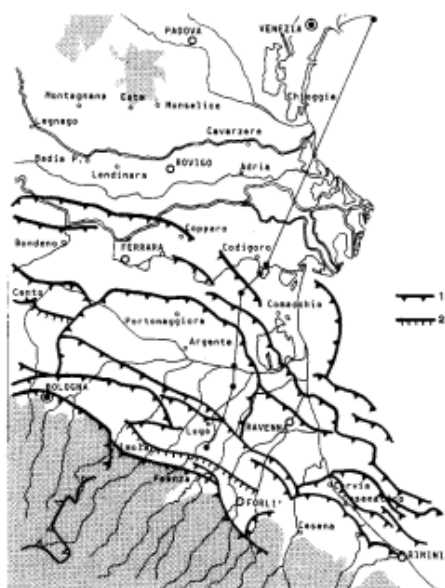
figura 2 - Principali strutture del substrato della Padania orientale, con l'Appennino sepolto:
