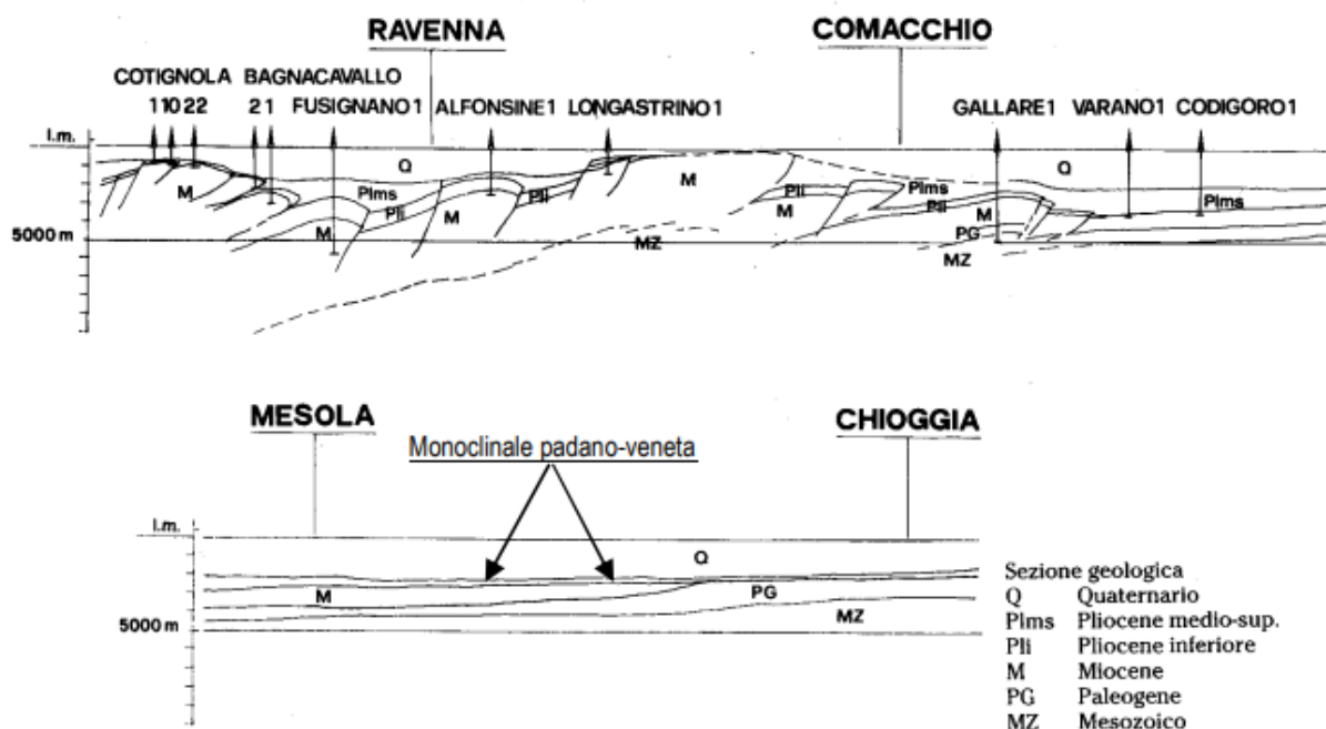
Figura 5 - Inquadramento geologico strutturale dell'area deltizia
