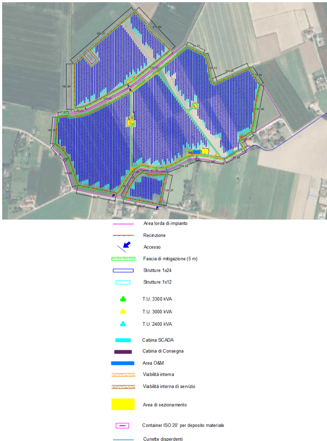
Figura 2 - Inquadramento su base ortofoto del layout di impianto
