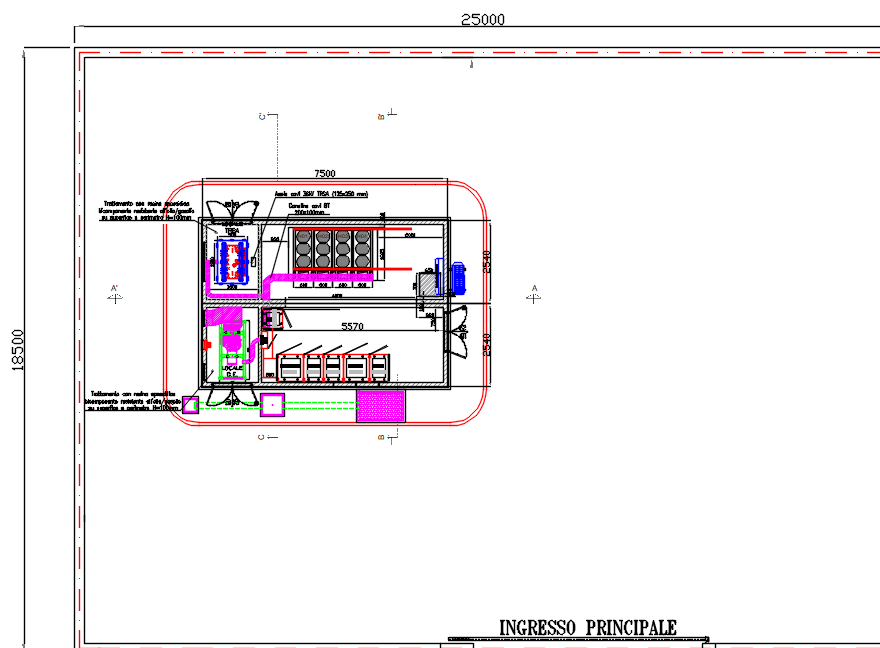
Figura 6 - Layout in pianta dell'area di sezionamento
