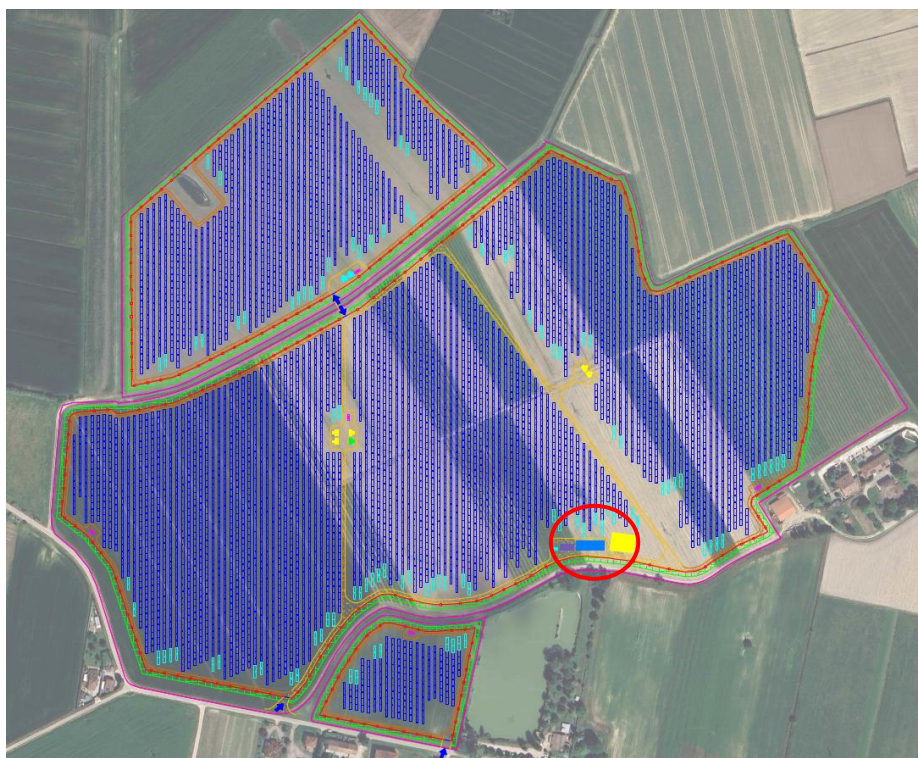
Figura 3 - Inquadramento su base ortofoto del layout di impianto con evidenza dell'area di sezionamento.
