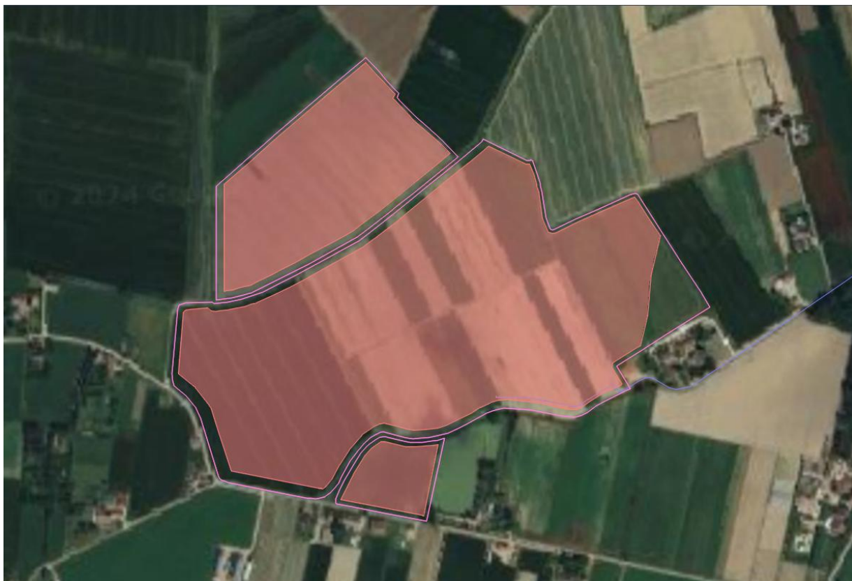
Figura 1 - Inquadramento su base ortofoto dell'area di impianto (in rosso) e dell'area di progetto (in magenta). In blu il cavidotto di connessione alla RTN
