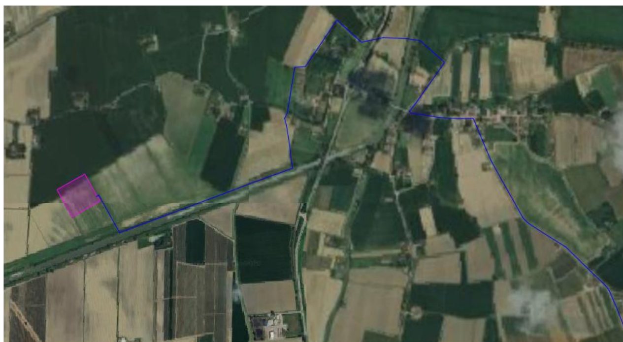
Figura 4 - Inquadramento su base ortofoto delle opere in progetto. In rosso l'area di impianto; in blu il cavidotto 36 kV; in magenta il futuro ampliamento della SE Terna.
