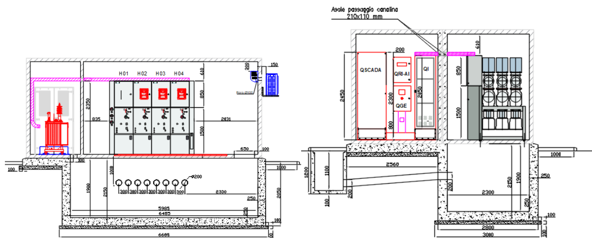
Figura 7 - sezione dei cabinati previsti per il sezionamento
