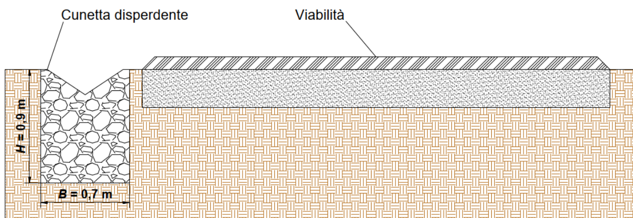
Figura 96 – Sezione tipologica della cunetta disperdente
