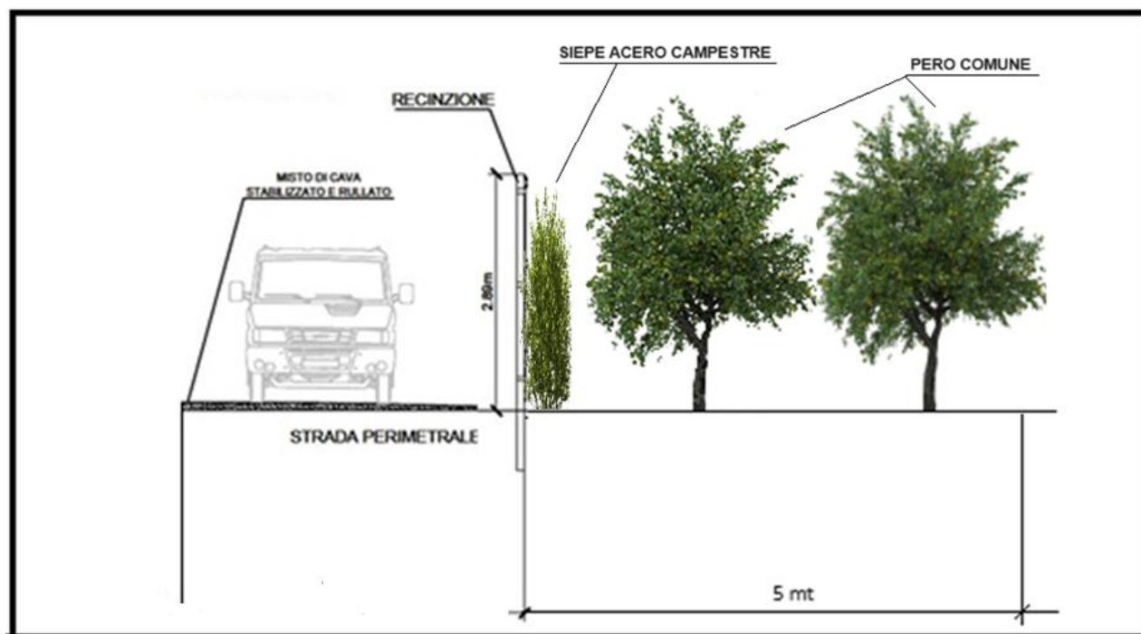
Figura 53 - Sezione della fascia di mitigazione rafforzata costituita da due file di peri da frutto in sesto a quinconce di 4x4 mt e una siepe in acero campestre
