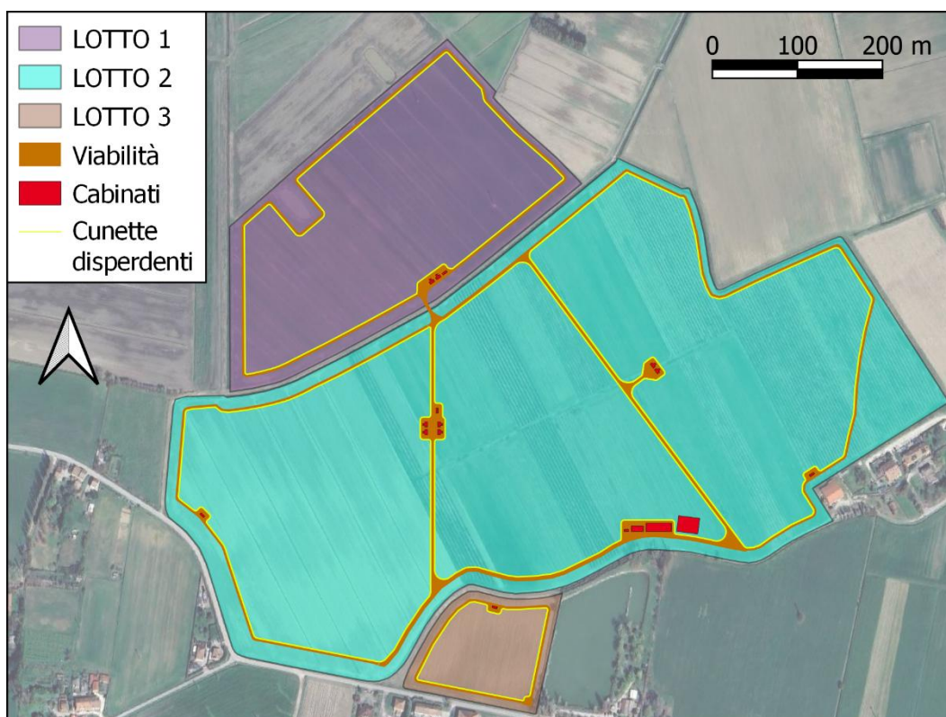
Figura 47 – Tracciato planimetrico delle cunette disperdenti
