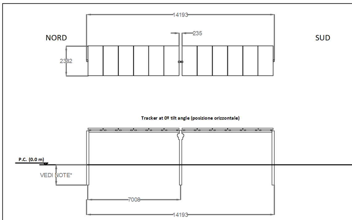
Figura 55 – Struttura tracker 1x12
