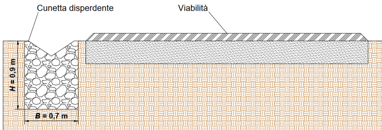
Figura 48 – Sezione tipologica della cunetta disperdente
