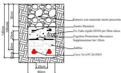
Figura 56 - Tipologico di posa cavidotti di impianto
