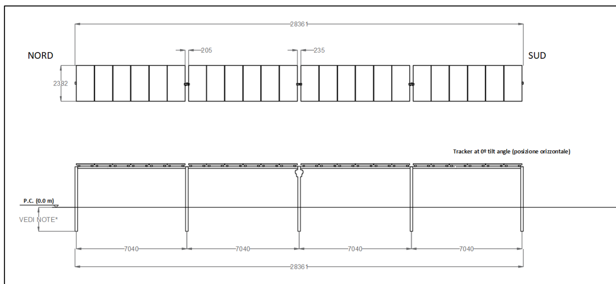
Figura 54 – Struttura tracker 1x24
