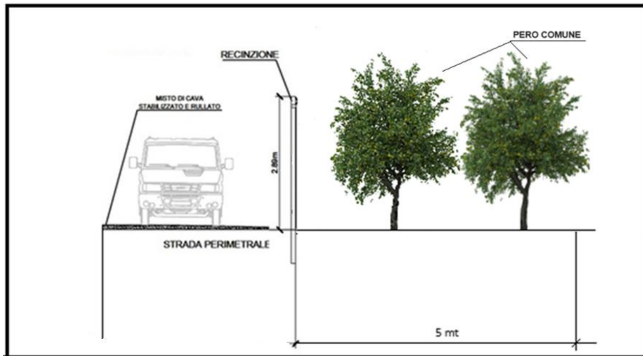
Figura 52 - Sezione della fascia di mitigazione normale costituita da due file di peri da frutto in sesto a quinconce di 4x4 mt
