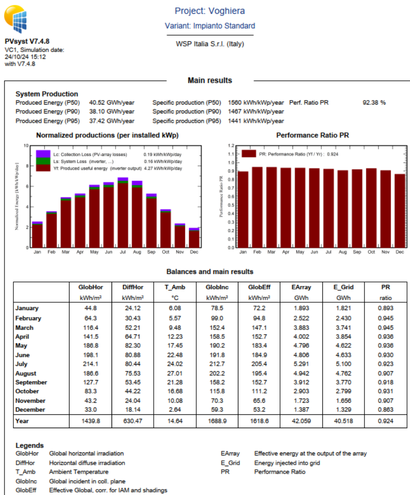
Figura 42 –Principali risultati relativi alla producibilità dell'impianto fotovoltaico standard.
