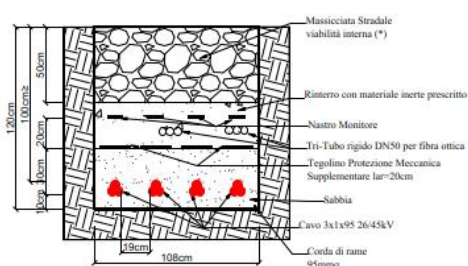
Figura 56 - Tipologico di posa cavidotti di impianto
