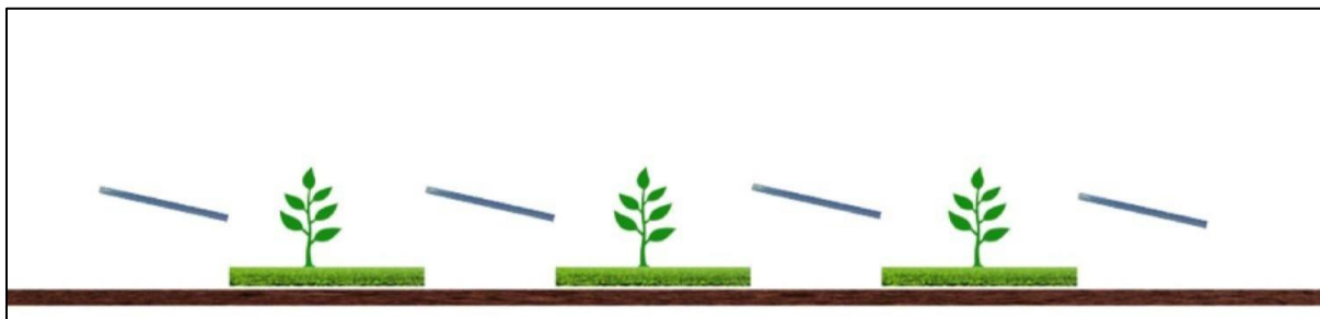
Figura 44- Sistema agrivoltaico avanzato in cui la coltivazione avviene tra le file dei moduli fotovoltaici, e non al di sotto di essi (TIPO 2).
