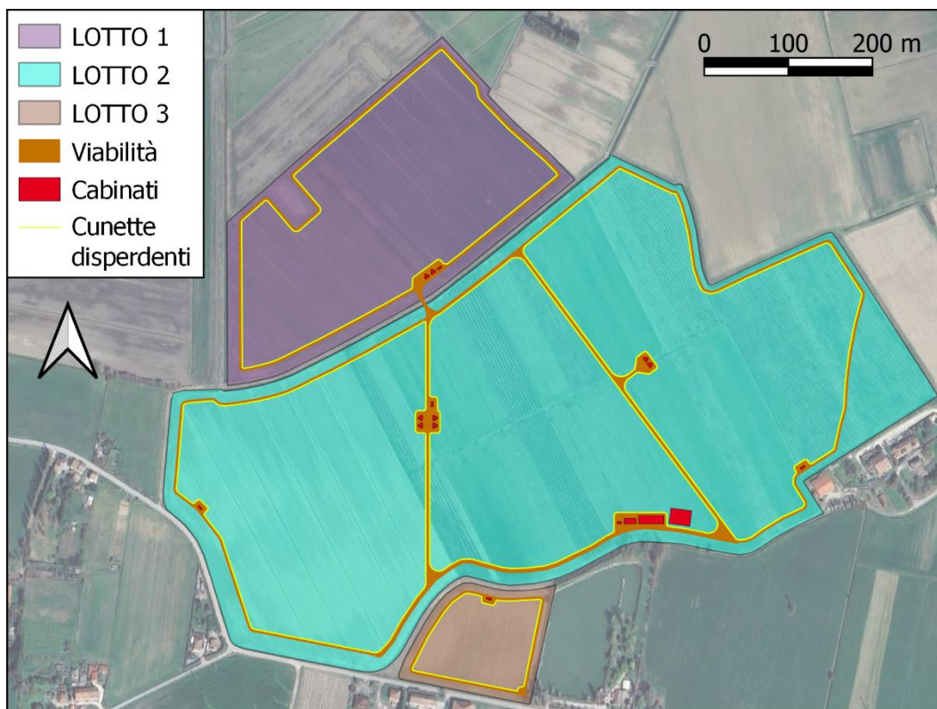
Figura 95 – Tracciato planimetrico delle cunette disperdenti
