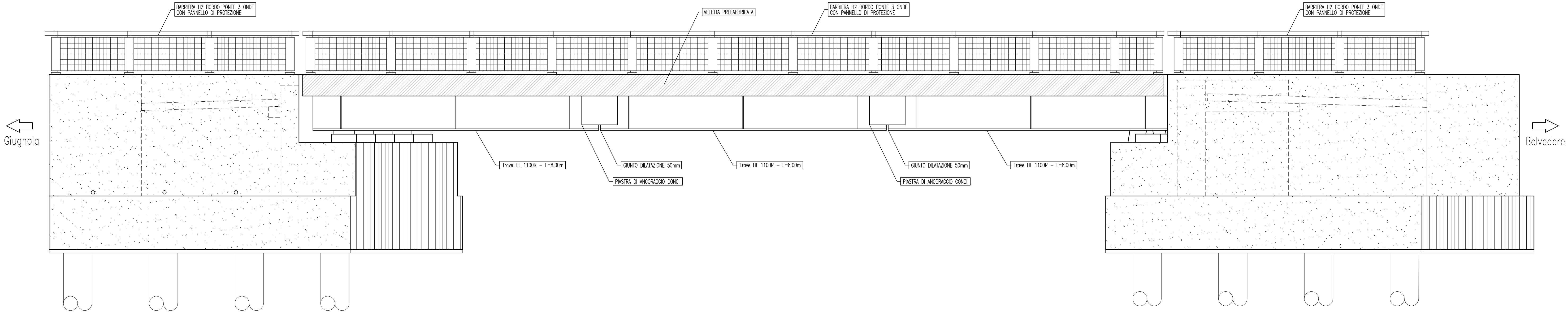
PROSPETTO LATO VALLE Scala 1:50
