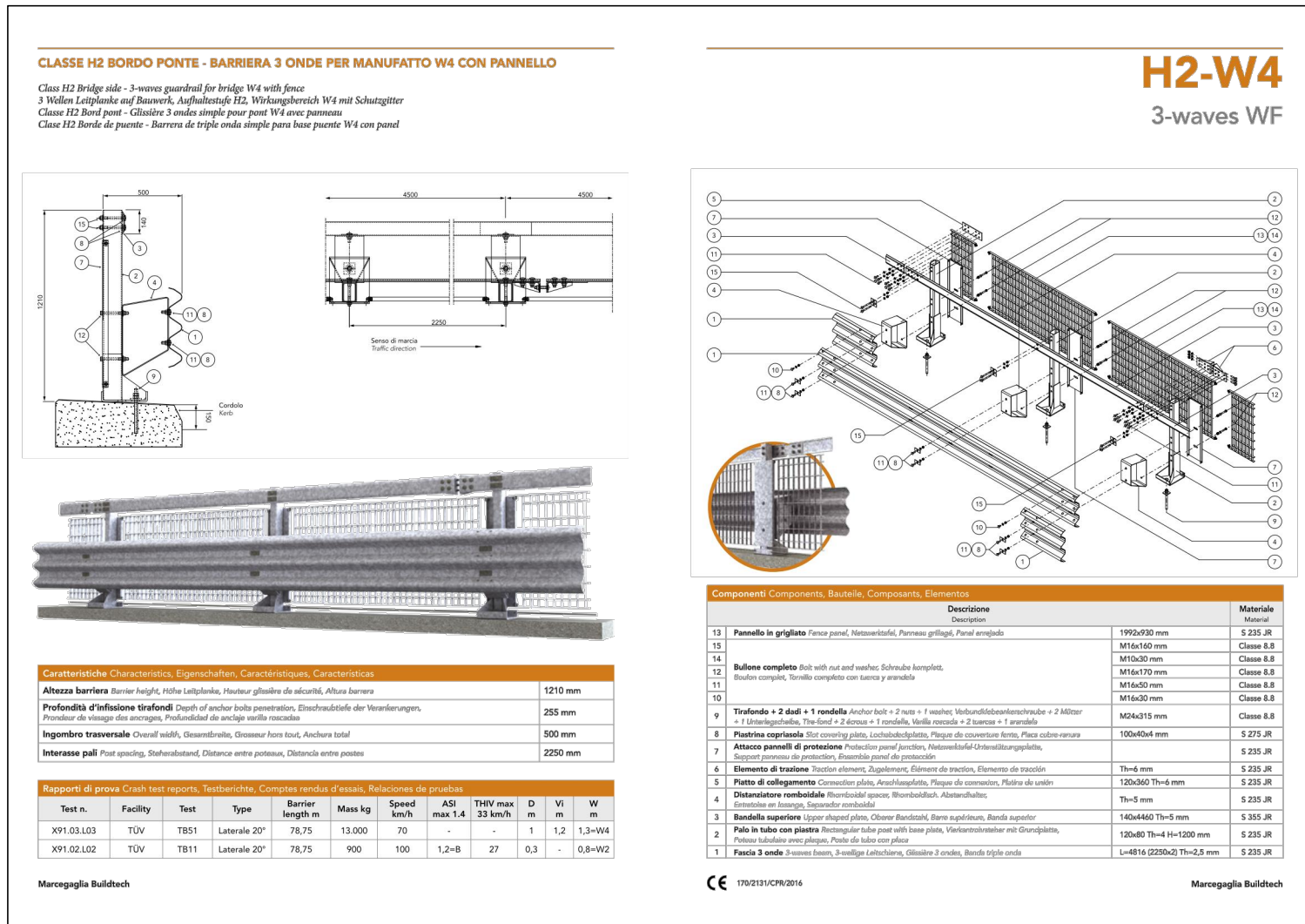
BARRIERA BORDO PONTE CON PANNELLO DI PROTEZIONE
