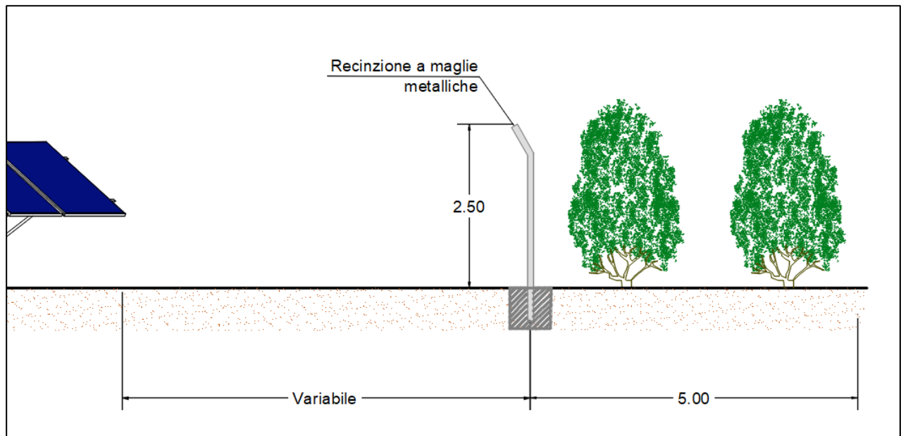
Figura 29 - Schematizzazione delle opere di mitigazione a verde
