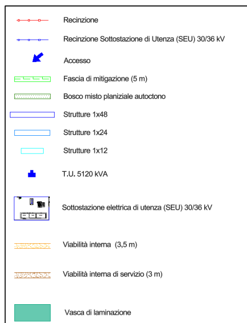
Figura 20 – Inquadramento su ortofoto del layout di impianto.
