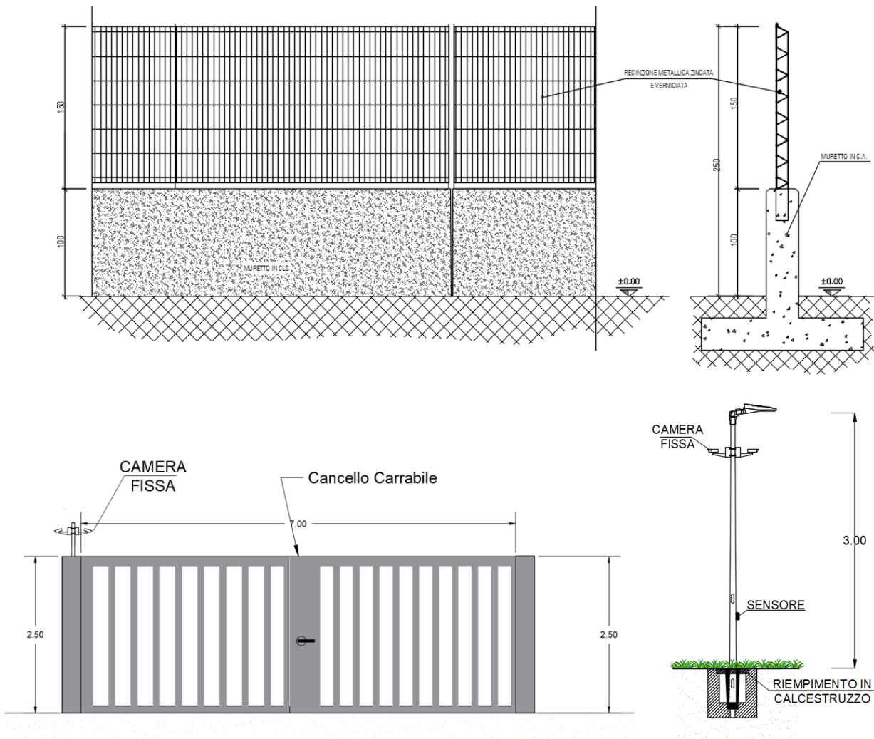
Figura 28 – Tipologici della recinzione, cancello e impianto di illuminazione e video sorveglianza previsti per l'area SEU.
