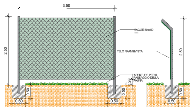
Figura 27 – Tipologici della recinzione con telo frangivista.
