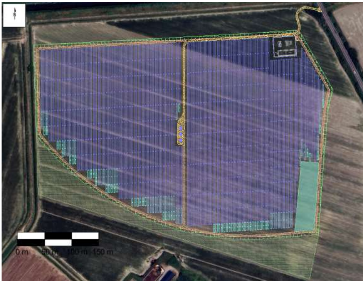
Figura 4 - Inquadramento su base ortofoto dell'area e del layout di impianto.
