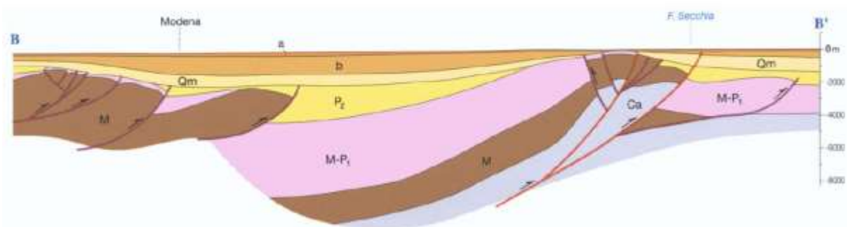
Figura 7 – Sezione geologica schematica dell'Appennino Reggiano
