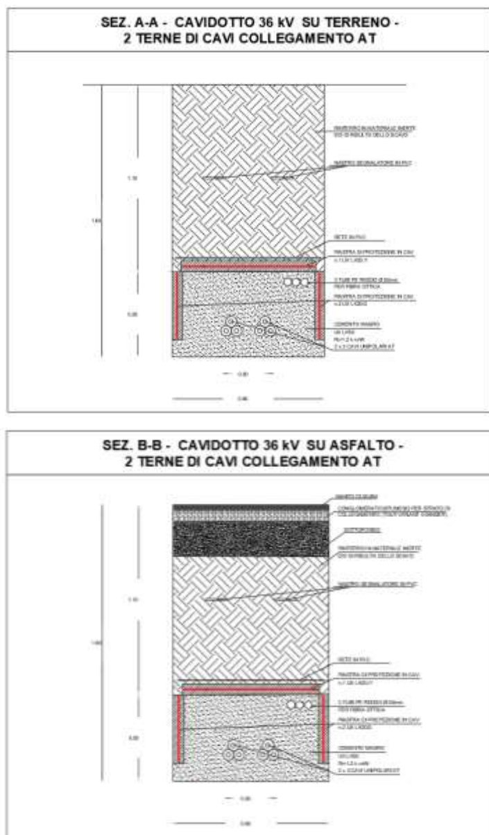
Figura 2: Tipologico di posa per il cavidotto AT interrato
