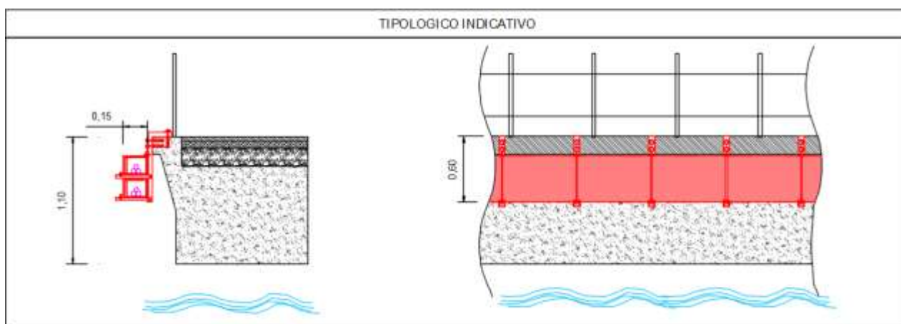
Figura 10 – Estratto elaborato “FAB.ENG.TAV.007.02_Planimetria delle interferenze” indicante un tipologico rappresentativo per il superamento dell’interferenza relativa all’attraversamento del corso idrico tutelato
