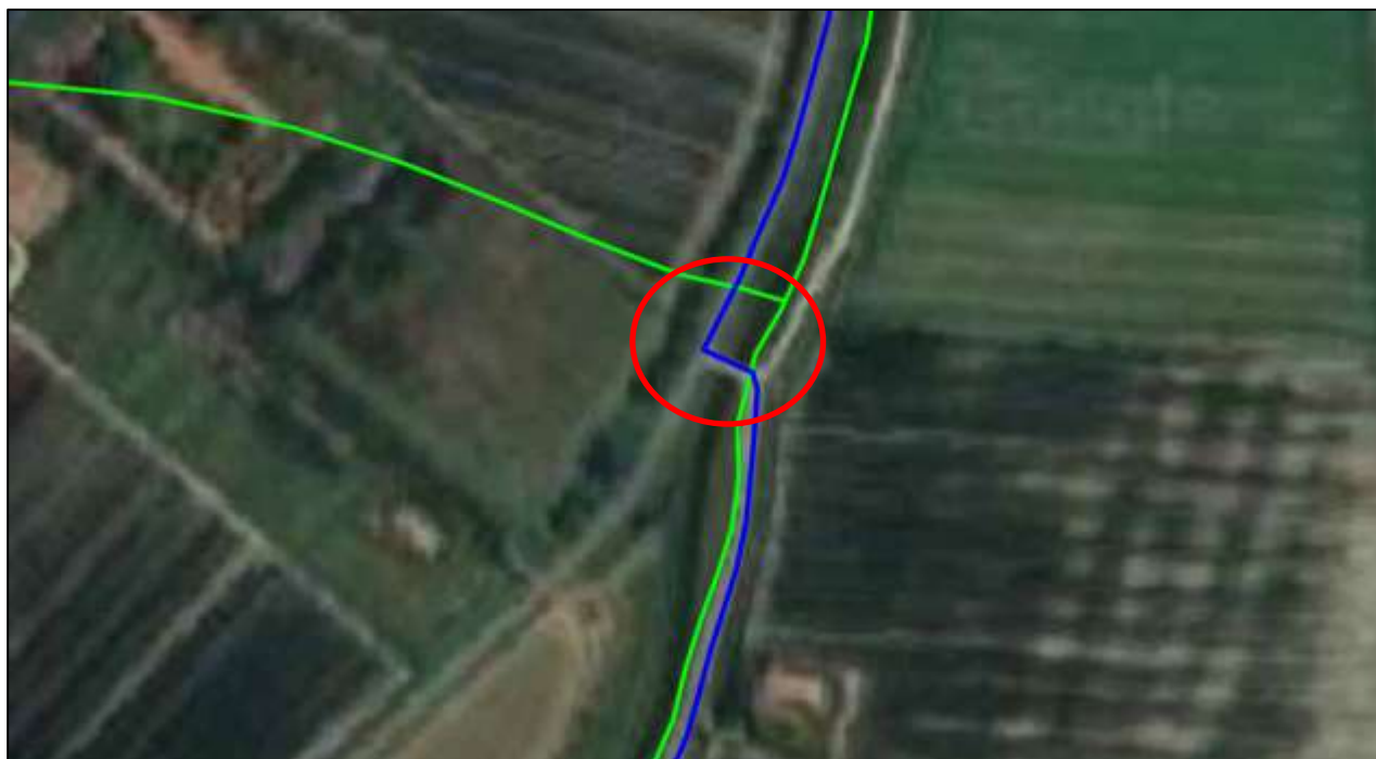
Figura 4: Estratto dell'elaborato "FAB.ENG.TAV.004.02_Inquadramento del progetto su ortofoto.pdf" rappresentante su ortofoto la sovrapposizione del cavidotto di connessione (in blu) che interessa l'attraversamento esistente (cerchio in rosso) sul fosso denominato "Fossa Raso e Tresinaro Vecchio" .
