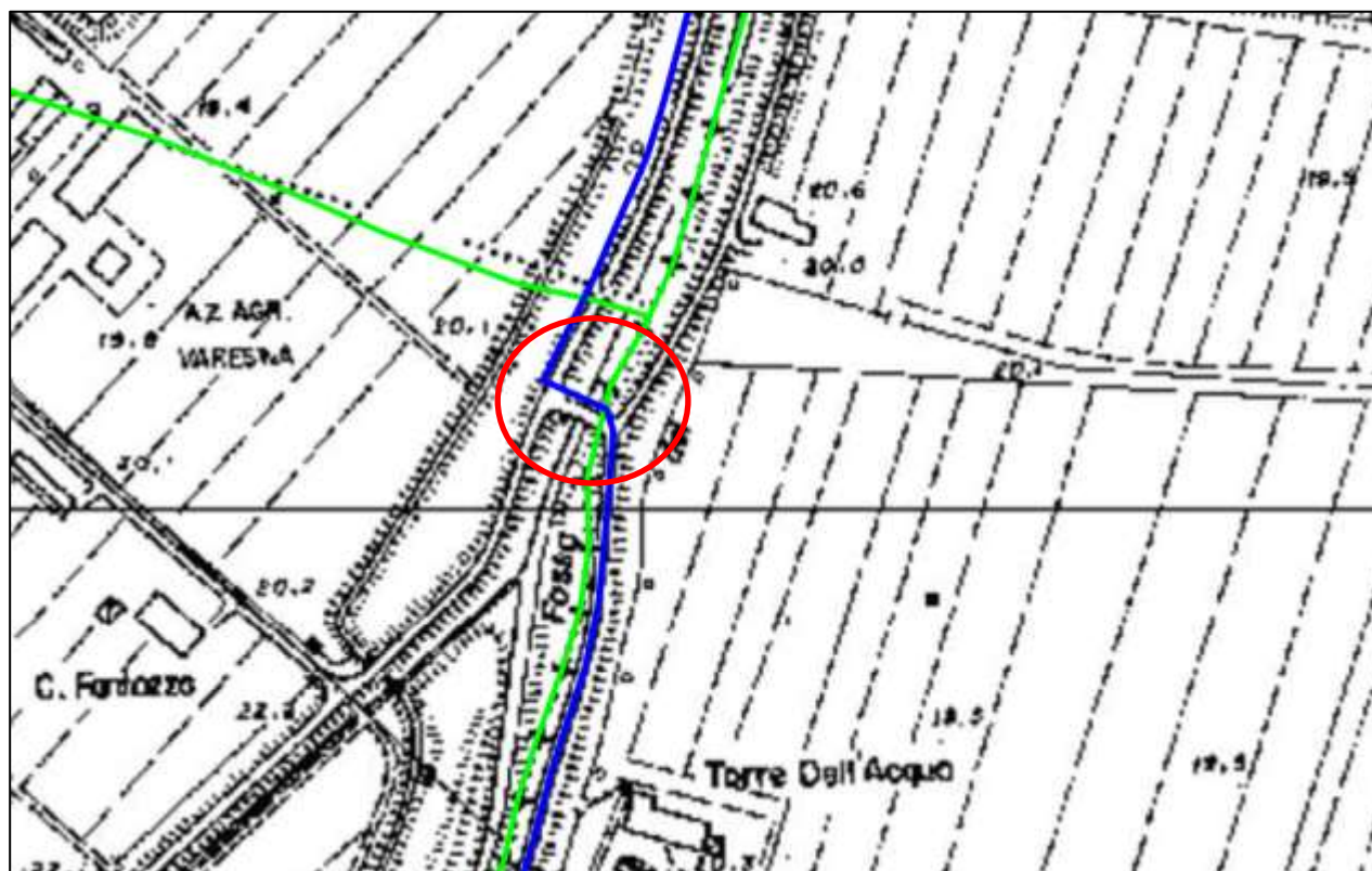
Figura 2: Estratto dell'elaborato "FAB.ENG.TAV.002.01_Inquadramento territoriale dell'intervento su base carta tecnica regionale, scala 1_10000.pdf" rappresentante su Carta Tecnica Regionale la sovrapposizione del cavidotto di connessione (in blu) che interessa l'attraversamento esistente (cerchio in rosso) sul fosso denominato "Fossa Raso e Tresinaro Vecchio". In verde i limiti comunali.
