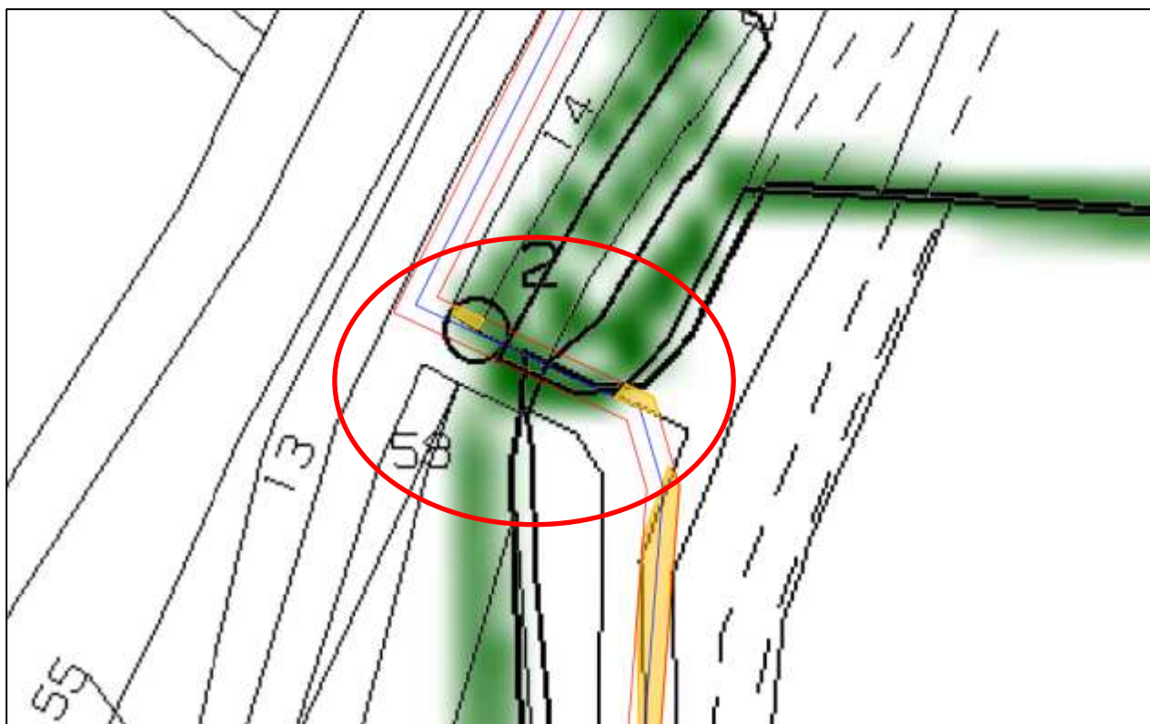
Figura 1: Estratto dell'elaborato "FAB.ENG.TAV.030.03_Inquadramento catastale opere di connessione alla rete.pdf" rappresentante la sovrapposizione su foglio catastale del cavidotto di connessione (in blu), fascia di asservimento (in rosso) e superficie di asservimento (in arancio) che interessa l'attraversamento esistente (cerchio in rosso) sul fosso denominato "Fossa Raso e Tresinaro Vecchio".
