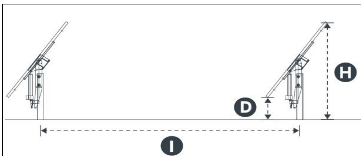
Figura 4: Profilo inseguitori monoassiali Est-Ovest
