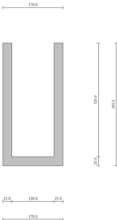
Figura 1 – Sezione canale in progetto
